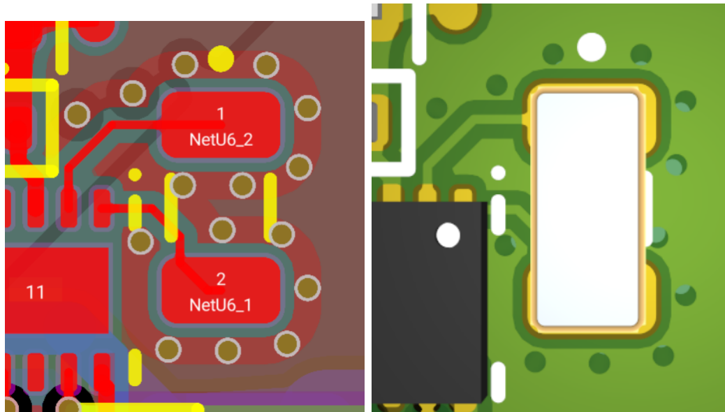
Hình 4.39: Kỹ thuật tạo vòng bảo vệ (Guard Ring) và via stitching xung quanh khối thạch anh để cô lập nhiễu.
