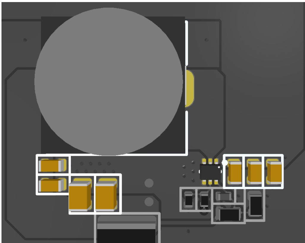
Hình 4.42: Vị trí các tụ điện trong nguồn xung +5V0_SYS.
