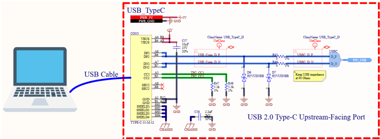
Hình 4.17: Sơ đồ nguyên lý mạch USB
