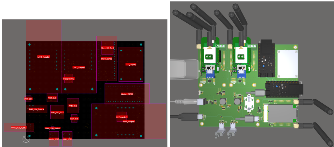
Hình 4.38: Sơ đồ quy hoạch phân vùng chức năng trên PCB (Floor-planning)
