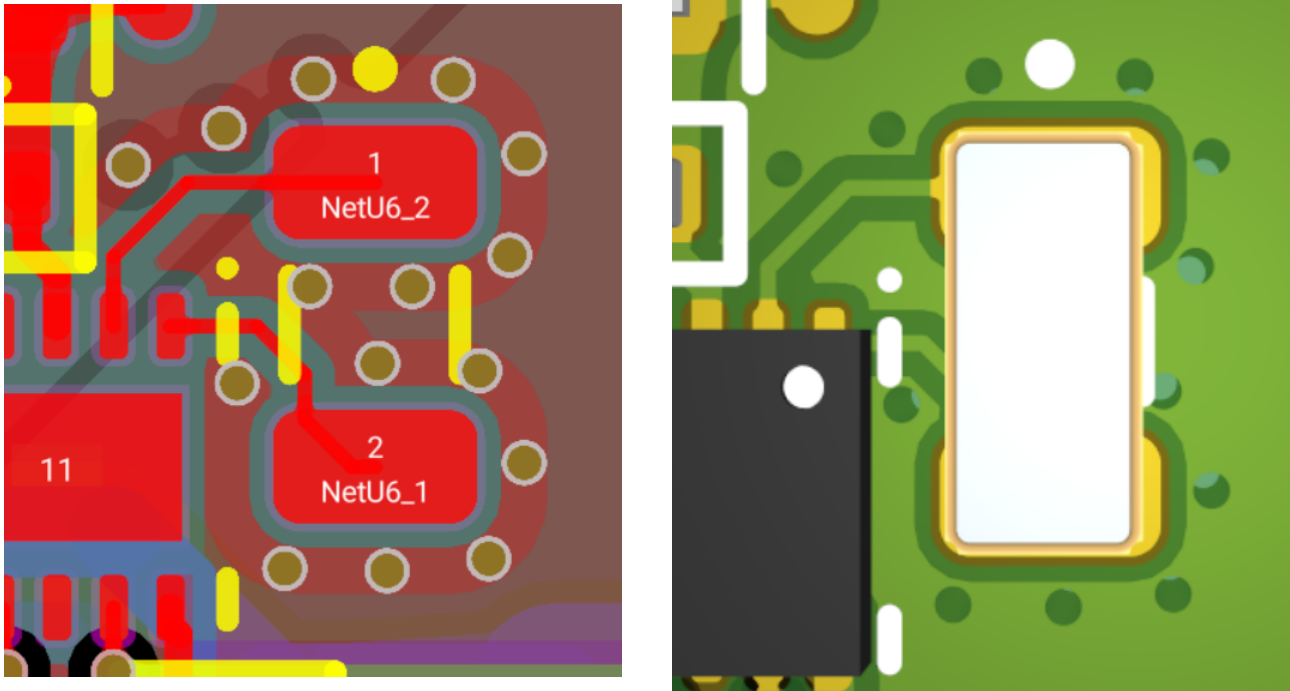
Hình 4.24: Kỹ thuật tạo vòng bảo vệ (Guard Ring) và via stitching xung quanh khối thạch anh để cô lập nhiễu.
