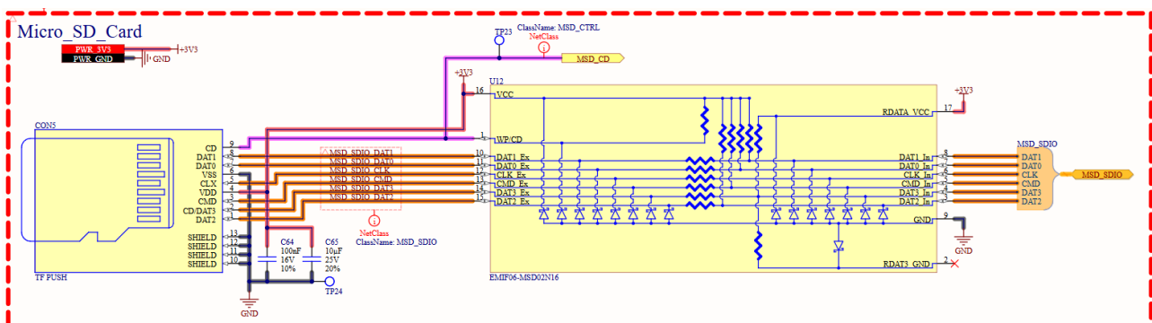
Hình 4.16: Sơ đồ nguyên lý mạch Micro SD Card
