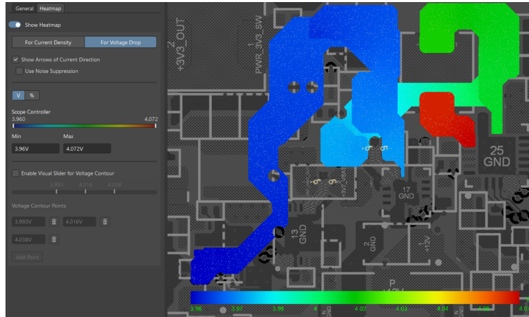
Hình 4.55: Biểu đồ phân bố điện áp (Voltage Drop Heatmap) trên nguồn +4V2_VSYS.
