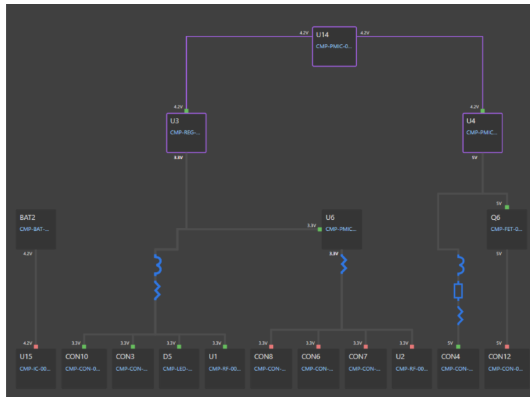
Hình 4.54: Cấu trúc mạng phân phối nguồn.
