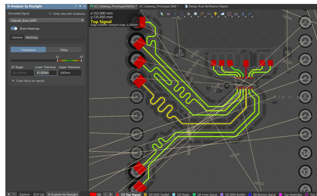
Hình 4.39: Biểu đồ phân bố trở kháng (Impedance Heatmap) đường tín hiệu đơn cực.
