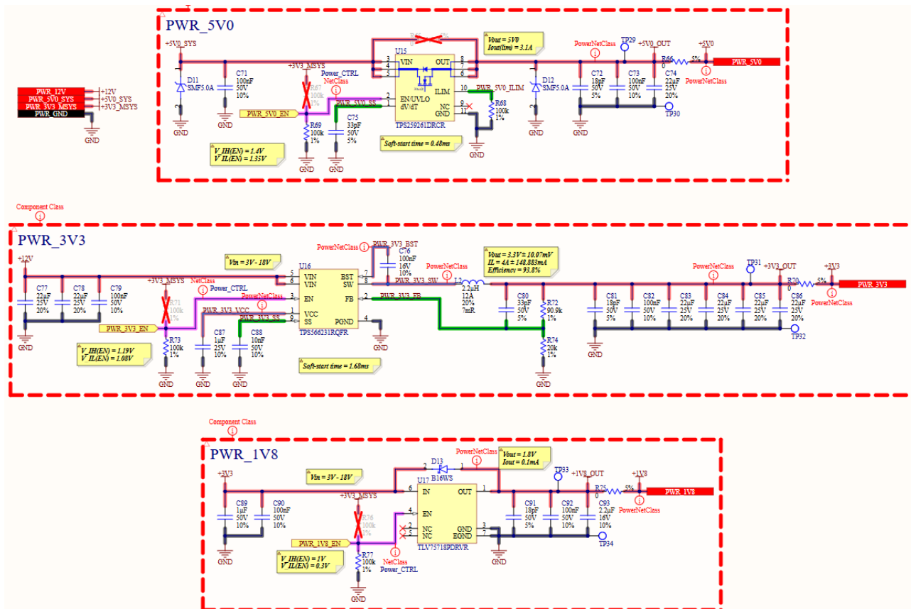
Hình 4.13: Sơ đồ nguyên lý mạch nguồn 2
