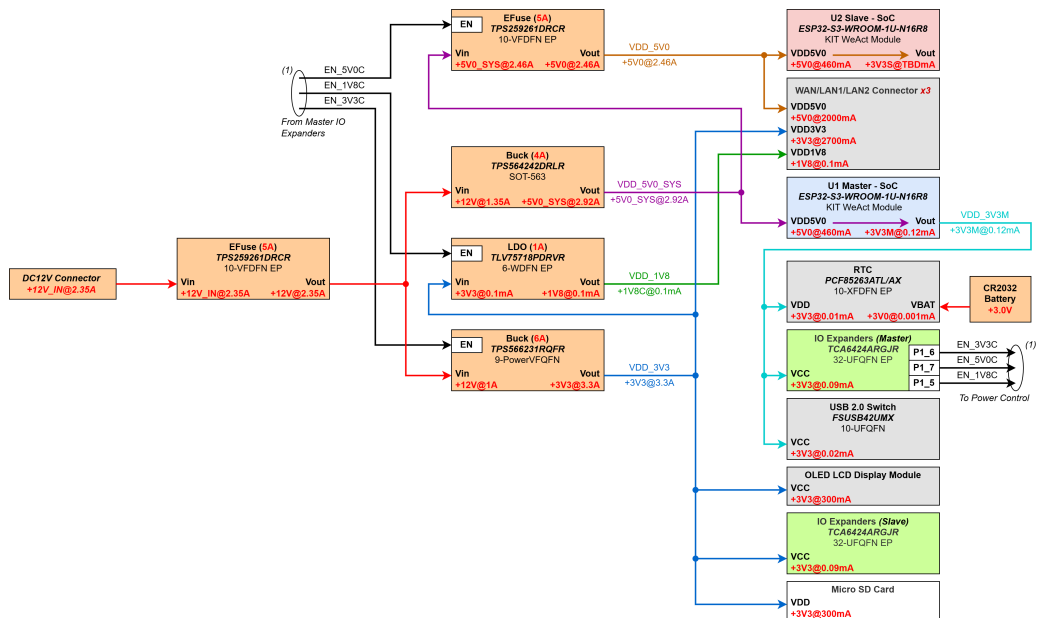
Hình 4.4: Sơ đồ khối nguồn
