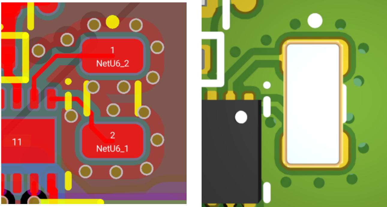
Hình 4.12: Kỹ thuật tạo vòng bảo vệ (Guard Ring) và via stitching xung quanh khối thạch anh để cô lập nhiễu.
