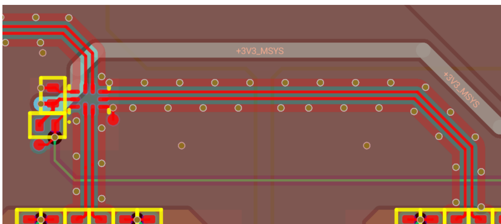
Hình 4.13: Kỹ thuật bọc mass và stitching via dọc theo đường tín hiệu USB tốc độ cao.
