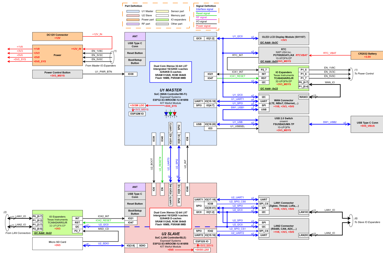
Hình 4.3: Sơ đồ khối Phần cứng
