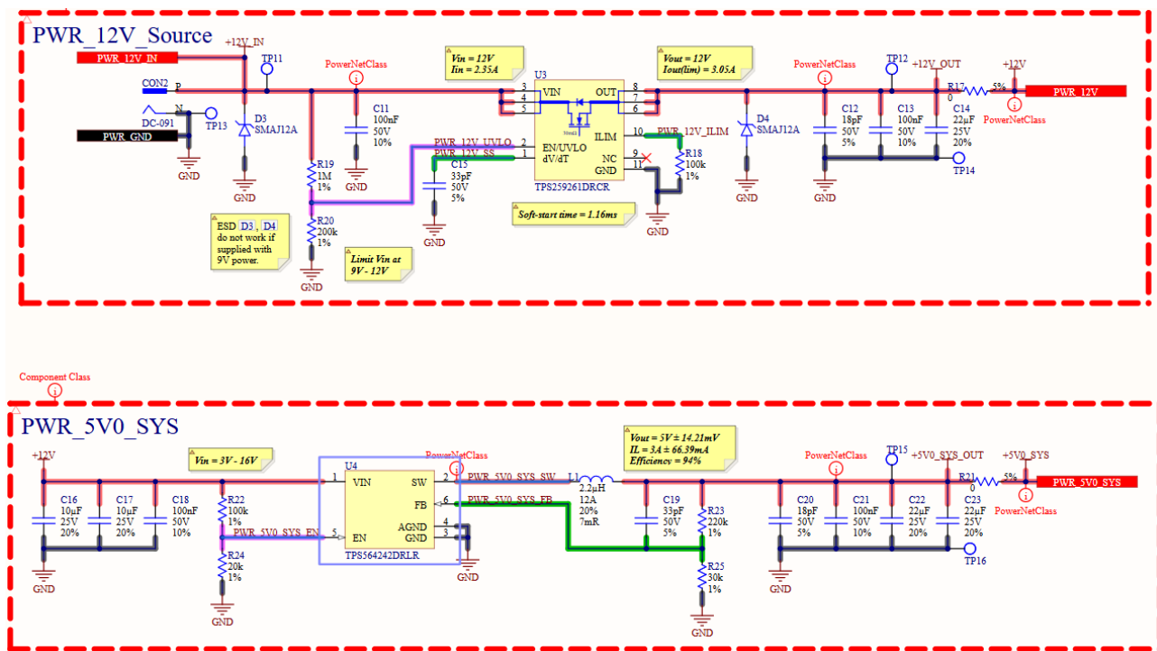
Hình 4.12: Sơ đồ nguyên lý mạch nguồn 1
