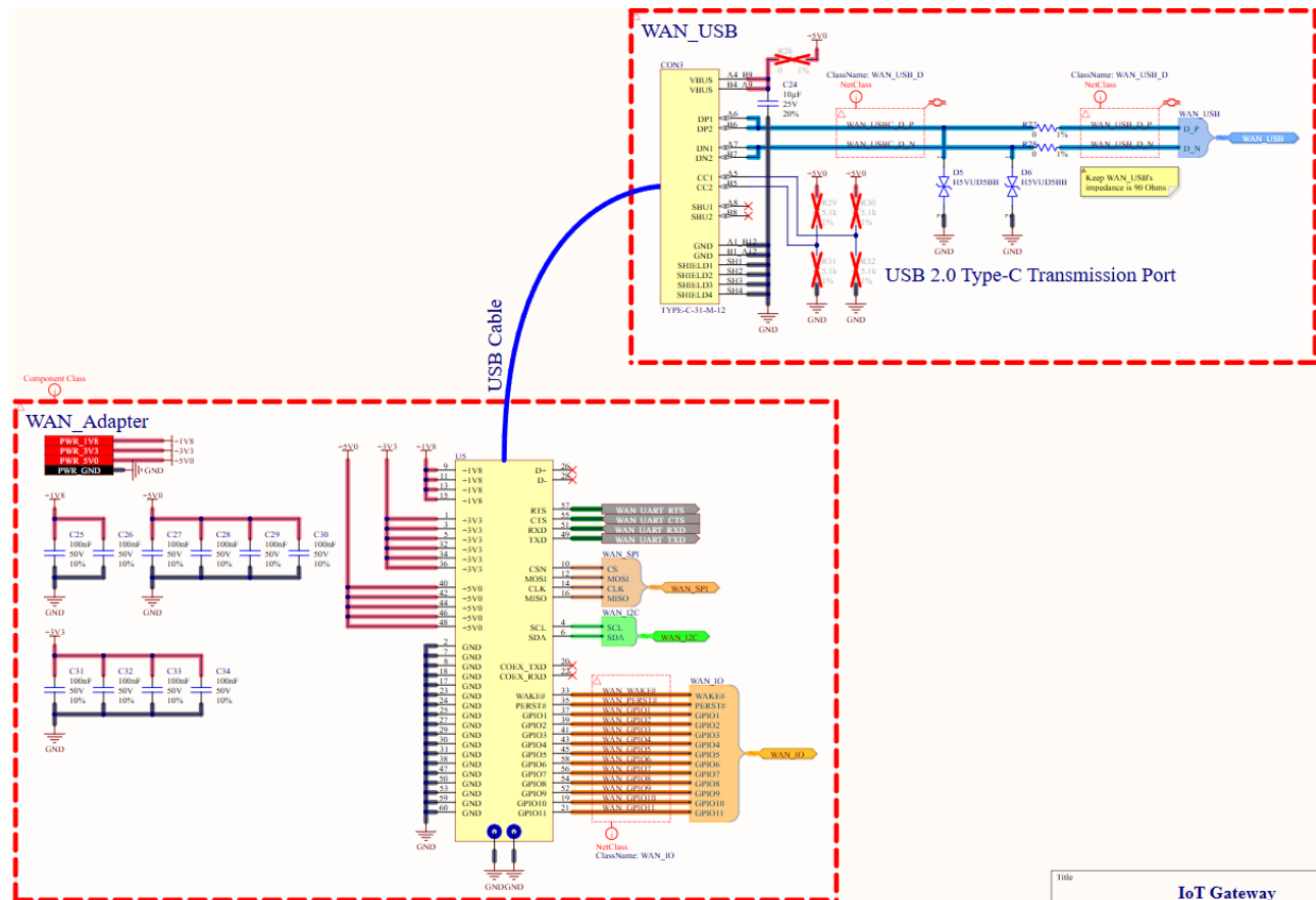
Hình 4.21: Sơ đồ nguyên lý mạch WAN
