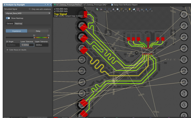
Hình 4.48: Biểu đồ phân bố trở kháng (Impedance Heatmap) đường tín hiệu đơn cực.
