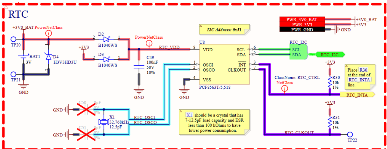
Hình 4.22: Sơ đồ nguyên lý mạch RTC
