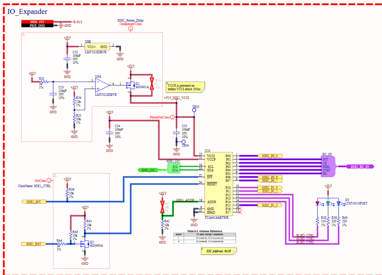
Hình 4.19: Sơ đồ nguyên lý mạch IO Expanders
