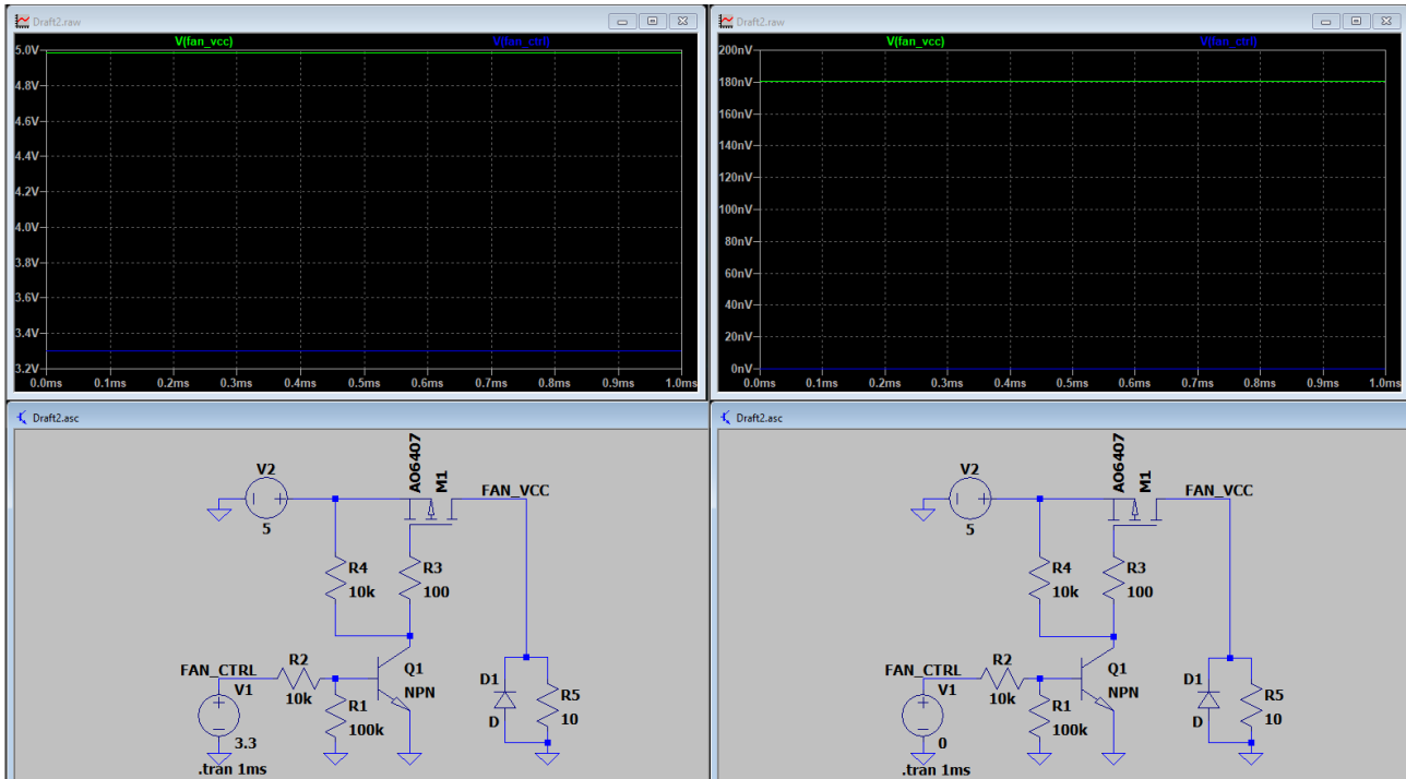
Hình 4.28: Thực hiện mô phỏng mạch điều khiển quạt DC trên LTspice
