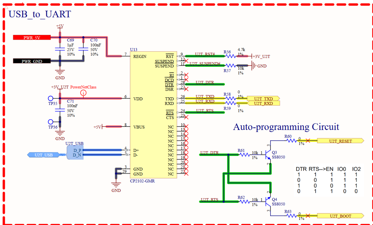
Hình 4.17: Sơ đồ nguyên lý mạch USB to UART Bridge
