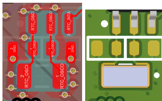
Hình 4.37: Kỹ thuật tạo vòng bảo vệ (Guard Ring) và via stitching xung quanh khối thạch anh để cô lập nhiễu.
