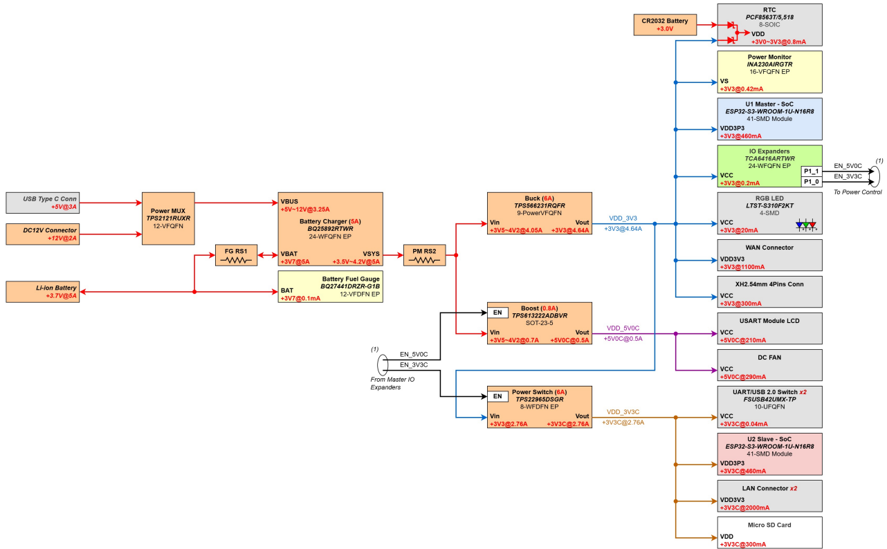
Hình 4.7: Sơ đồ hệ thống nguồn
