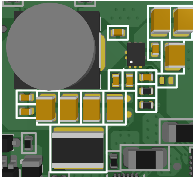
Hình 4.40: Vị trí các tụ điện trong nguồn xung +3V3.
