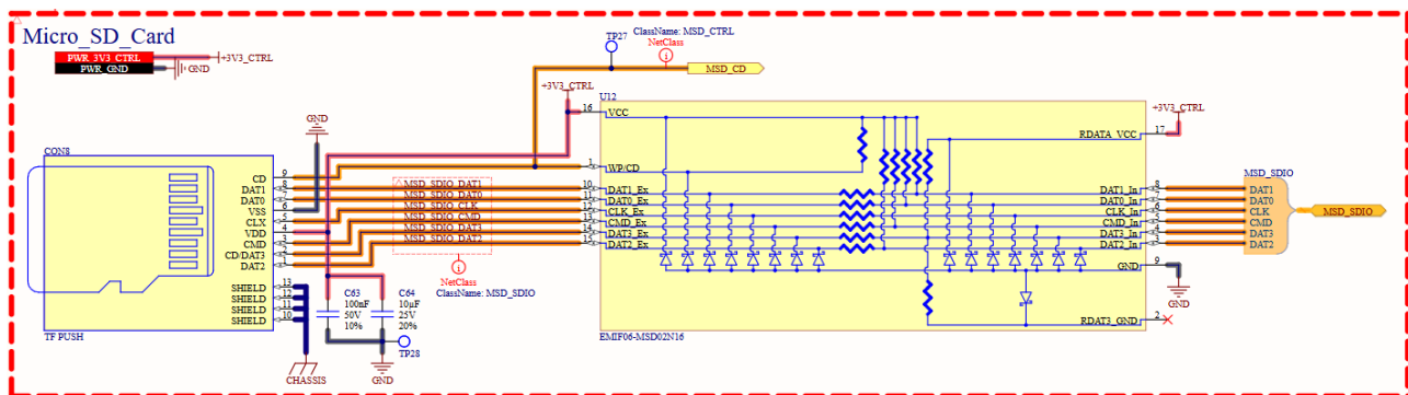
Hình 4.22: Sơ đồ nguyên lý mạch Micro SD Card
