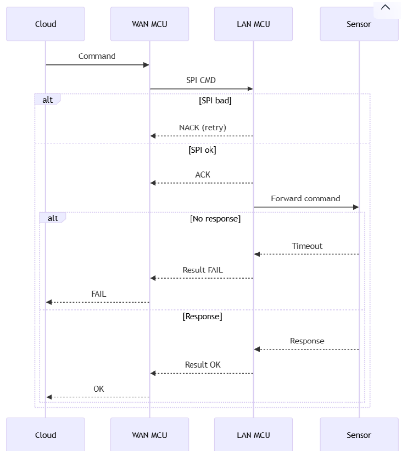
Hình 4.3: Sequence diagram: luồng xử lý dữ liệu end-to-end downlink
