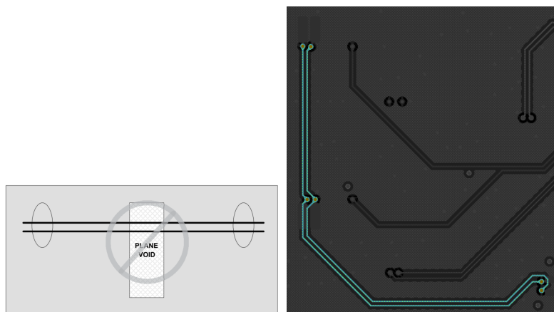
Hình 4.39: Minh họa tín hiệu Slave_I2C0 được định tuyến liên tục trên mặt phẳng GND đồng nhất, tránh các vị trí lớp phủ đã bị cắt.
