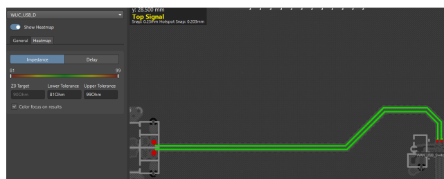
Hình 4.49: Biểu đồ phân bố trở kháng (Impedance Heatmap) đường vi sai.
