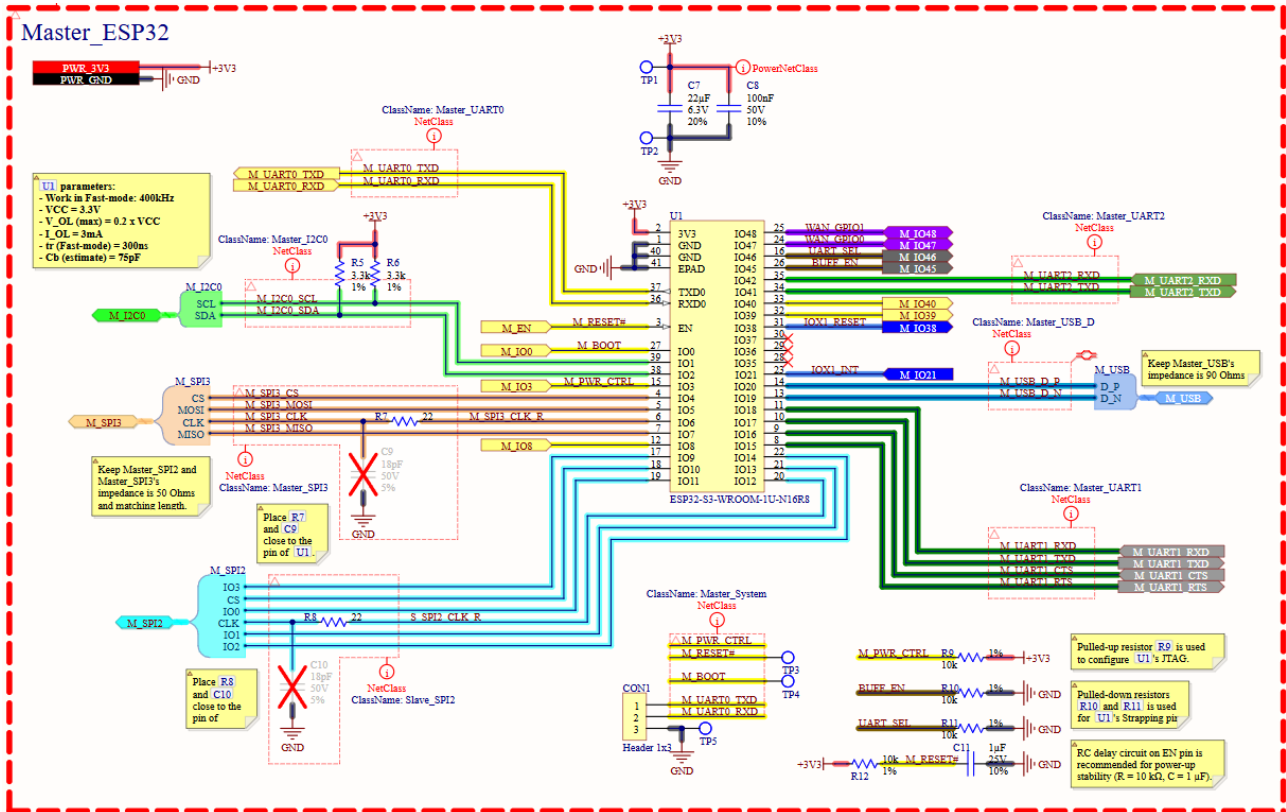
Hình 4.10: Sơ đồ nguyên lý ESP32 Master
