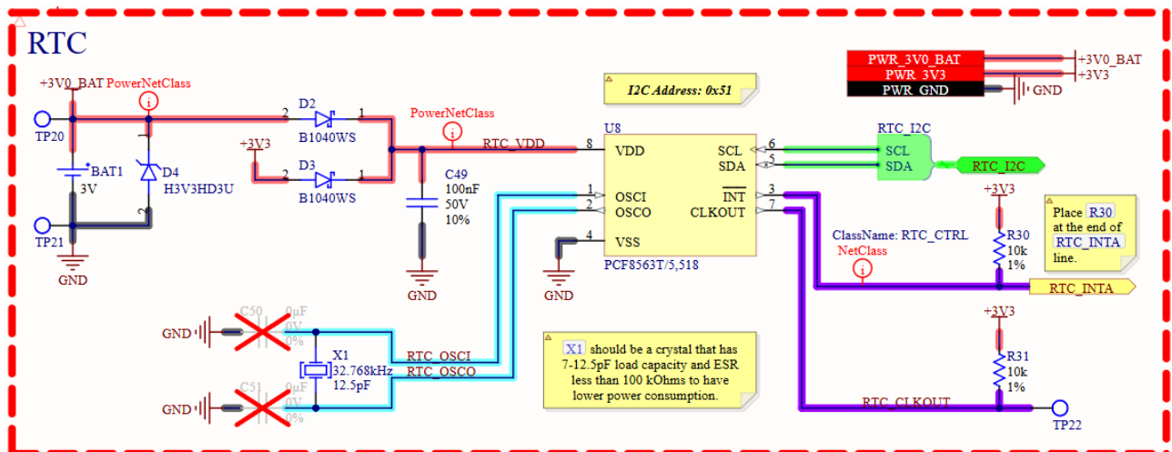
Hình 4.21: Sơ đồ nguyên lý mạch RTC
