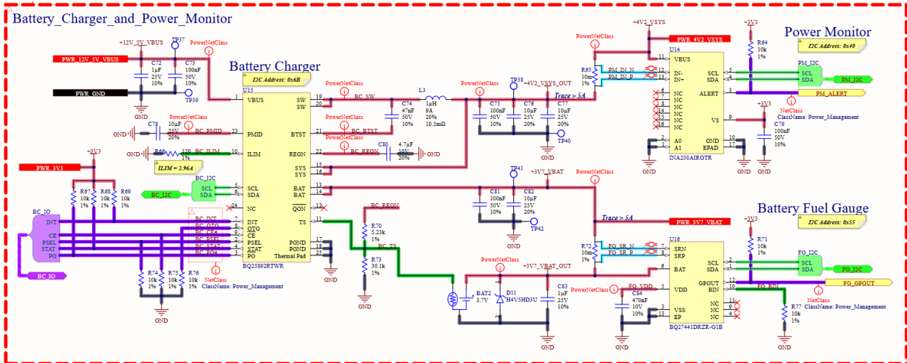
Hình 4.14: Sơ đồ nguyên lý mạch sạc, quản lý pin LiPo và giám sát công suất
