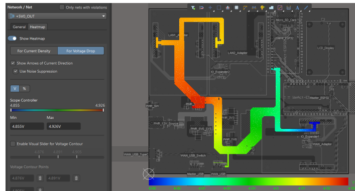
Hình 4.54: Biểu đồ phân bố điện áp (Voltage Drop Heatmap) trên nguồn +5V0.
