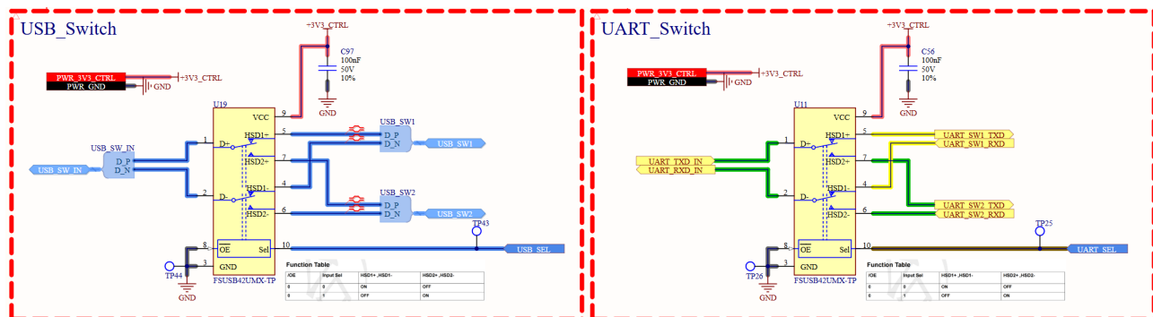
Hình 4.23: Sơ đồ nguyên lý mạch USB/UART Switch
