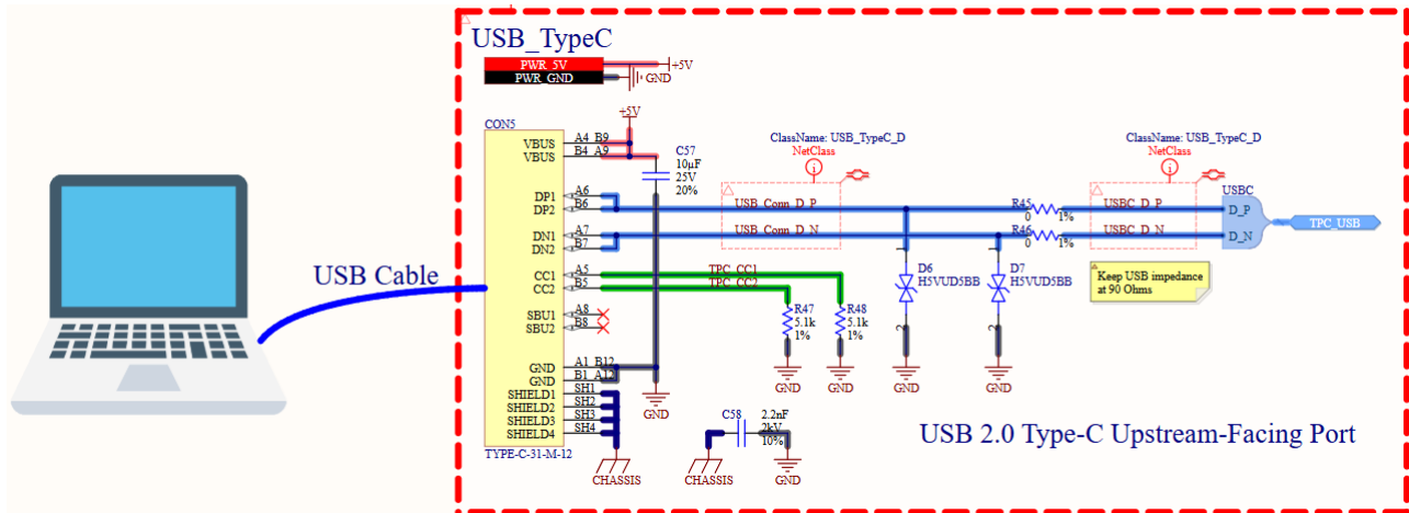
Hình 4.16: Sơ đồ nguyên lý mạch USB
