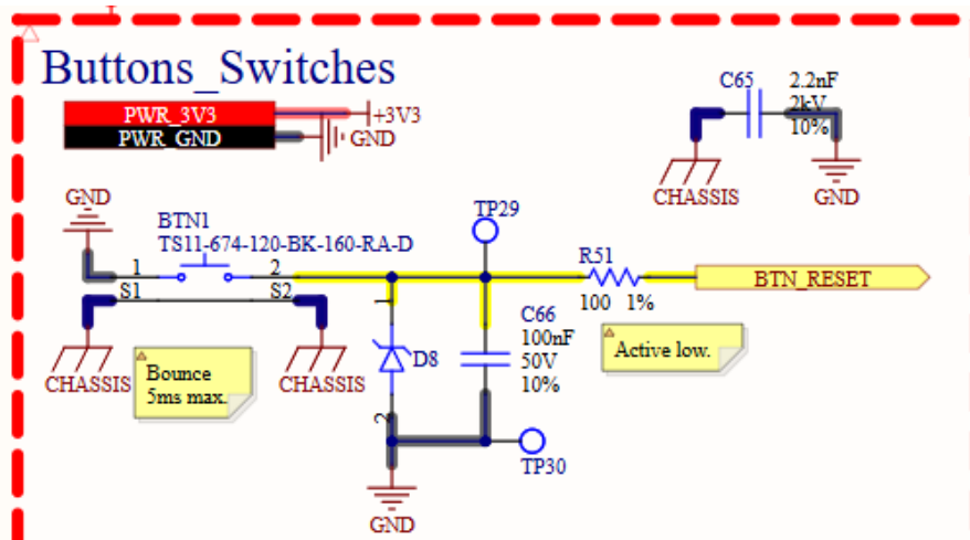
Hình 4.26: Sơ đồ nguyên lý mạch nút nhấn
