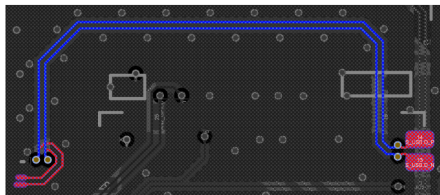
Hình 4.44: Định tuyến USB.
