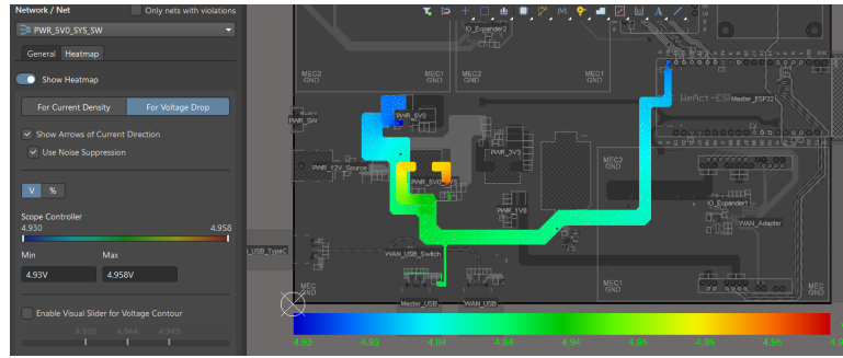
Hình 4.53: Biểu đồ phân bố điện áp (Voltage Drop Heatmap) trên nguồn +5V0_SYS.
