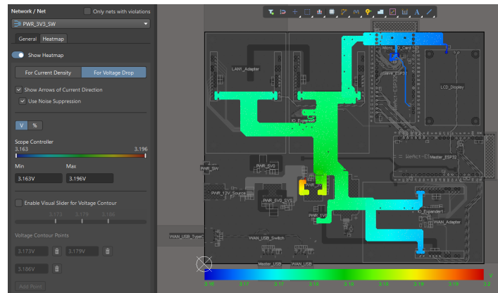
Hình 4.55: Biểu đồ phân bố điện áp (Voltage Drop Heatmap) trên nguồn +3V3.
