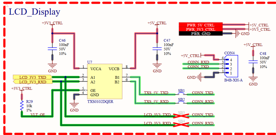
Hình 4.24: Sơ đồ nguyên lý mạch LCD
