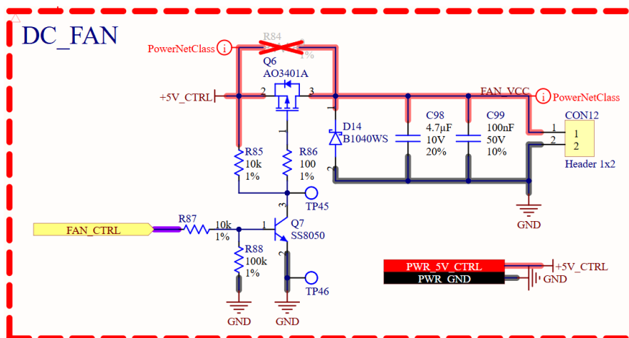
Hình 4.27: Sơ đồ nguyên lý mạch điều khiển quạt DC
