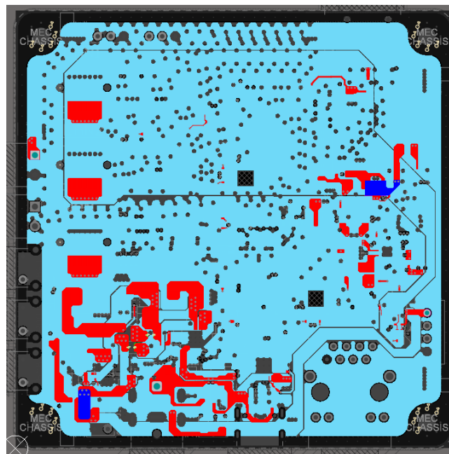
Hình 4.43: Mạng phân phối nguồn.
