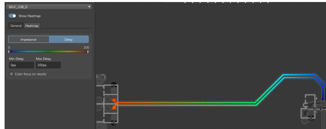
Hình 4.50: Biểu đồ phân bố độ trễ lan truyền (Propagation Delay) đường vi sai.
