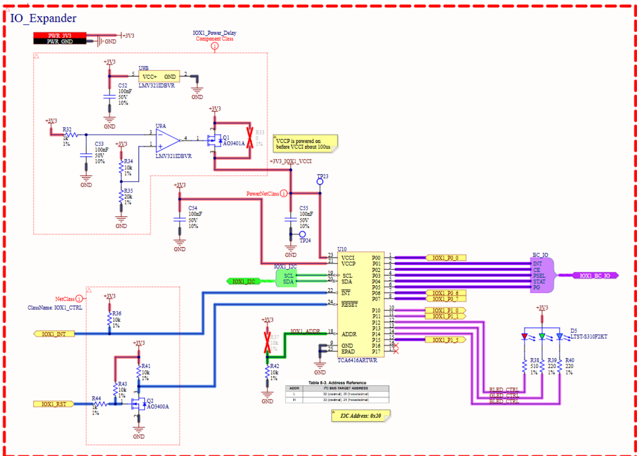
Hình 4.18: Sơ đồ nguyên lý mạch IO Expanders
