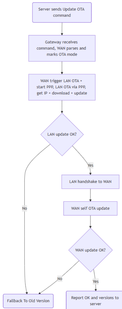
Hình 4.64: Lưu đồ giải thuật FOTA cho Dual-MCU Gateway
