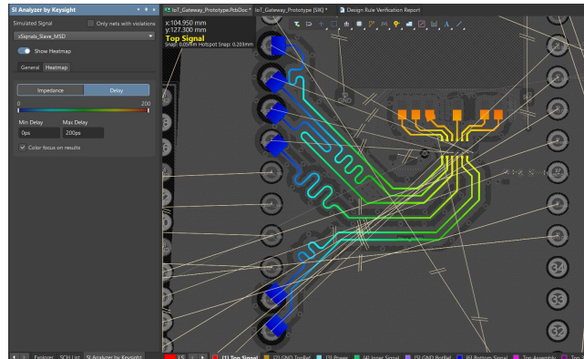
Hình 4.47: Biểu đồ phân bố độ trễ lan truyền (Propagation Delay) đường tín hiệu đơn cực.
