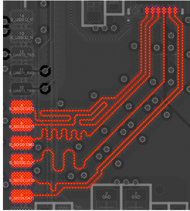
Hình 4.45: Định tuyến SDIO giữa ESP32-S3 Slave với Micro SD Card.
