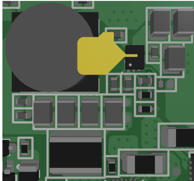
Hình 4.41: Điểm chuyển mạch trong nguồn xung +3V3.
