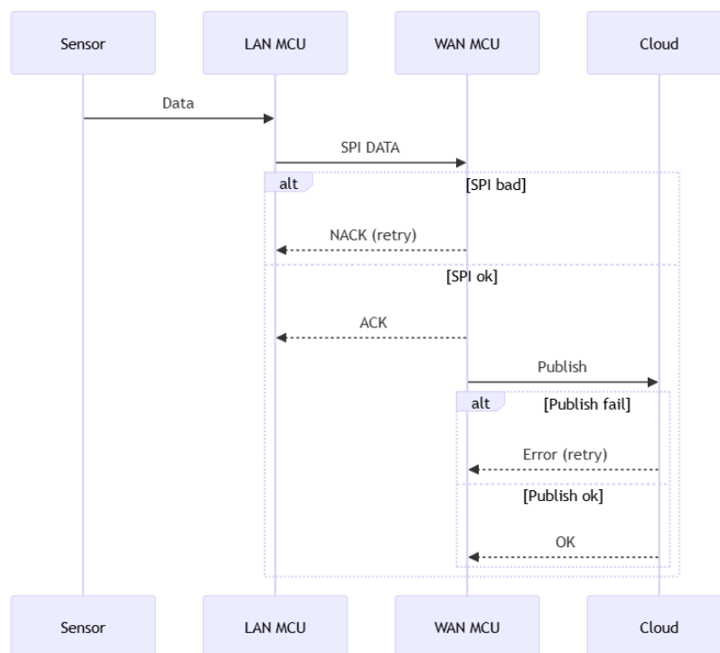
Hình 4.2: Sequence diagram: luồng xử lý dữ liệu end-to-end uplink
