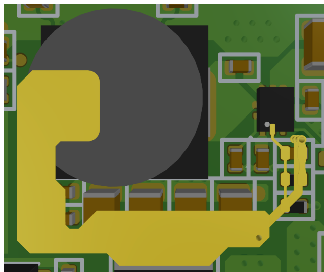
Hình 4.42: Định tuyến hồi tiếp trong nguồn xung +3V3.
