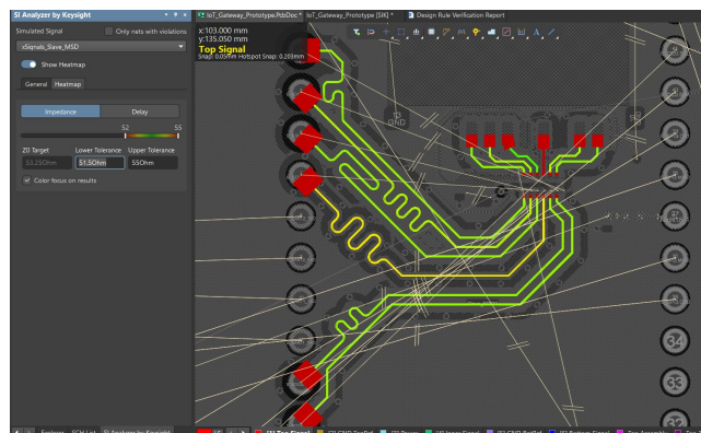
Hình 4.46: Biểu đồ phân bố trở kháng (Impedance Heatmap) đường tín hiệu đơn cực.
