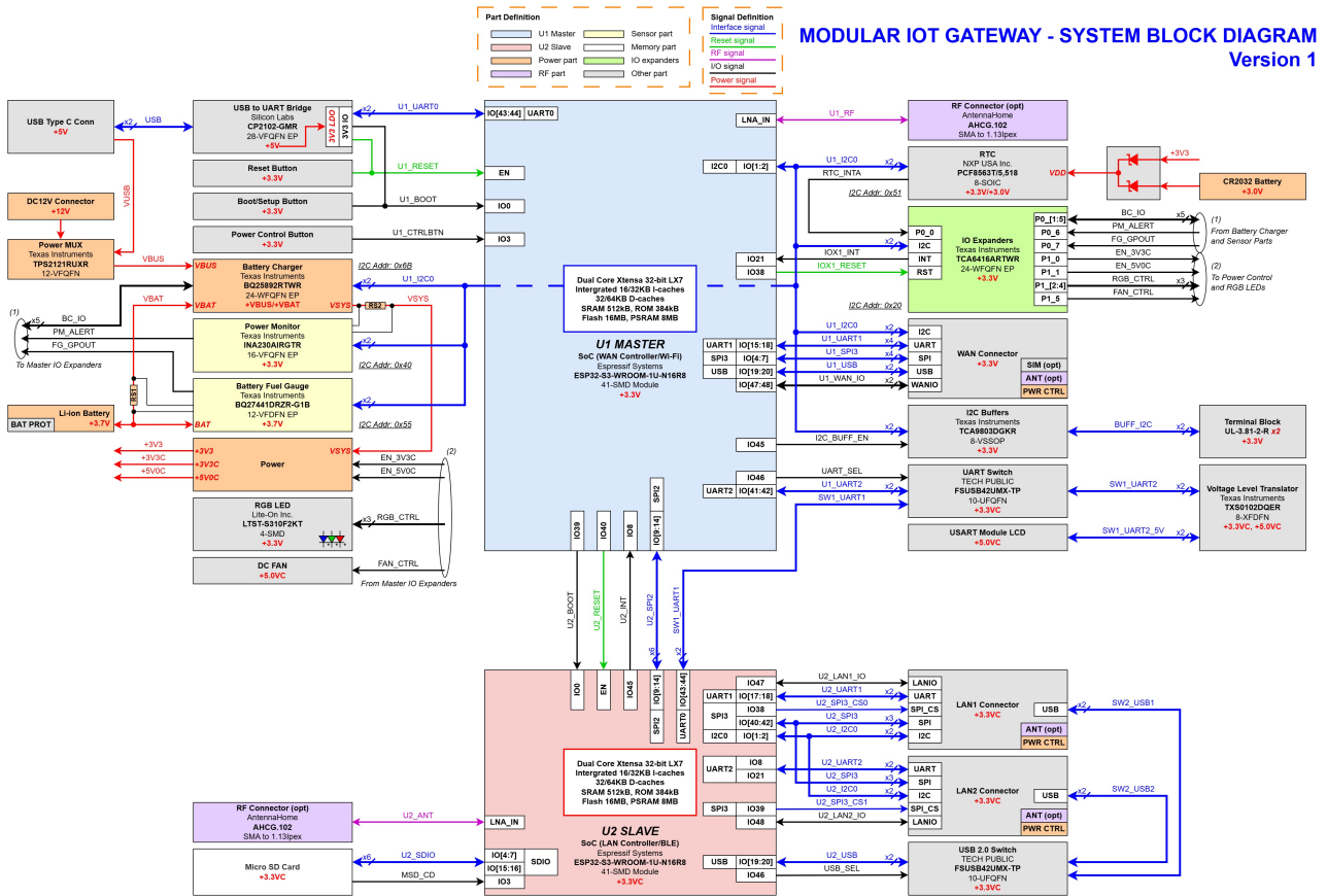
Hình 4.6: Sơ đồ khối hệ thống
