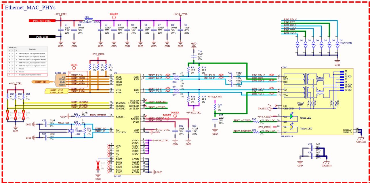
Hình 4.31: Sơ đồ nguyên lý mạch WAN Adapter Ethernet
