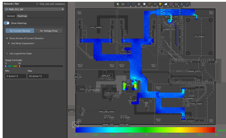
Hình 4.59: Biểu đồ phân bố mật độ dòng điện (Current Density Heatmap) trên nguồn +3V3.
