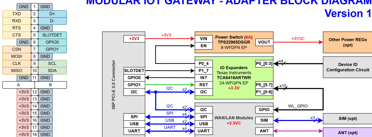
Hình 4.8: Sơ đồ khối mạch adapter
