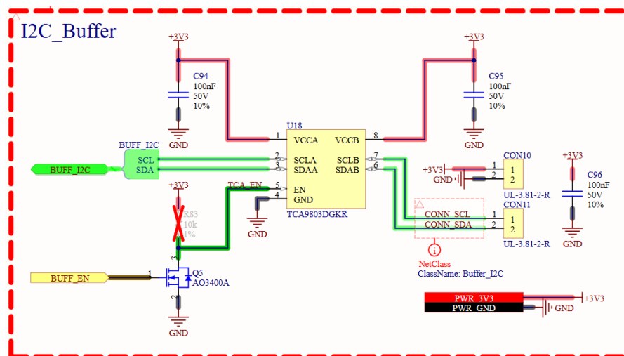
Hình 4.25: Sơ đồ nguyên lý mạch I 2 C Buffer
