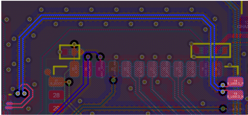
Hình 4.38: Kỹ thuật bọc mass và stitching via dọc theo đường tín hiệu USB tốc độ cao.
