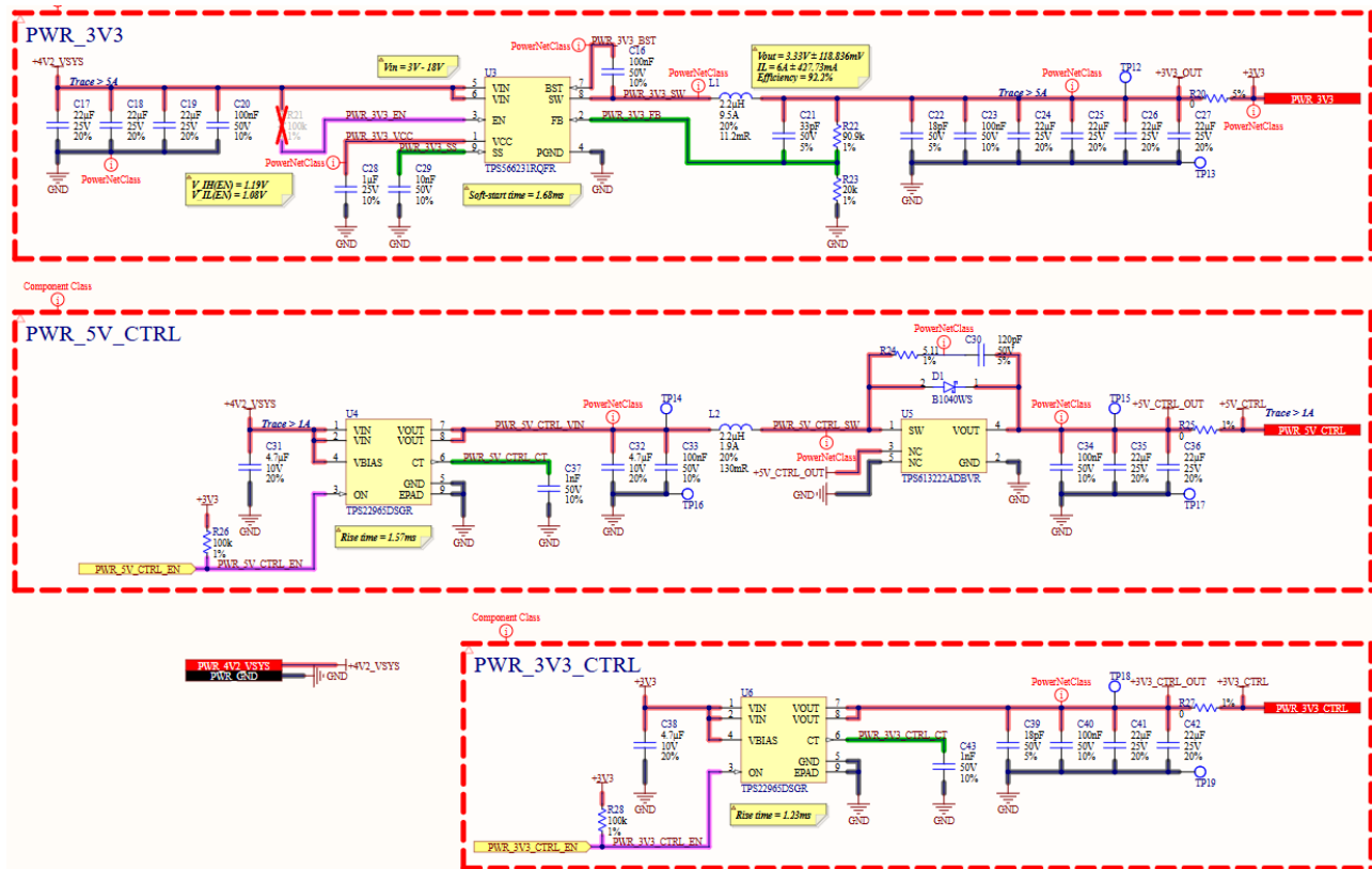
Hình 4.15: Sơ đồ nguyên lý mạch nguồn DC-DC
