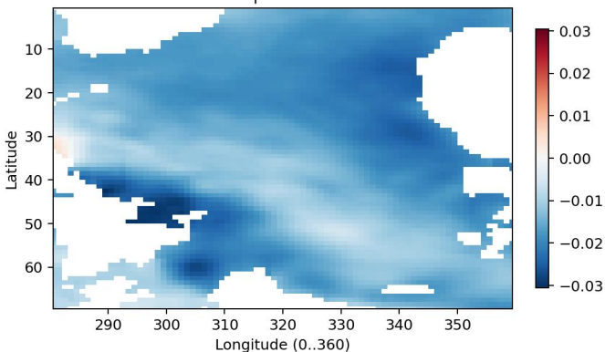
EOF3 | EVR=0.097
