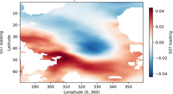
EOF6 | EVR=0.035
