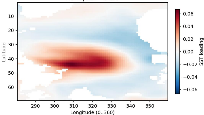
EOF5 | EVR=0.044
