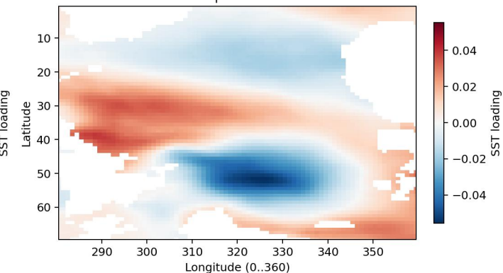
EOF4 | EVR=0.053
