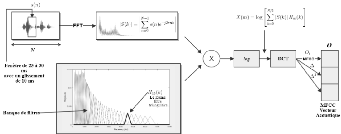
Figure 18 : processus d'extraction d'un vecteur MFCC à partir d'une trame de parole [44]
