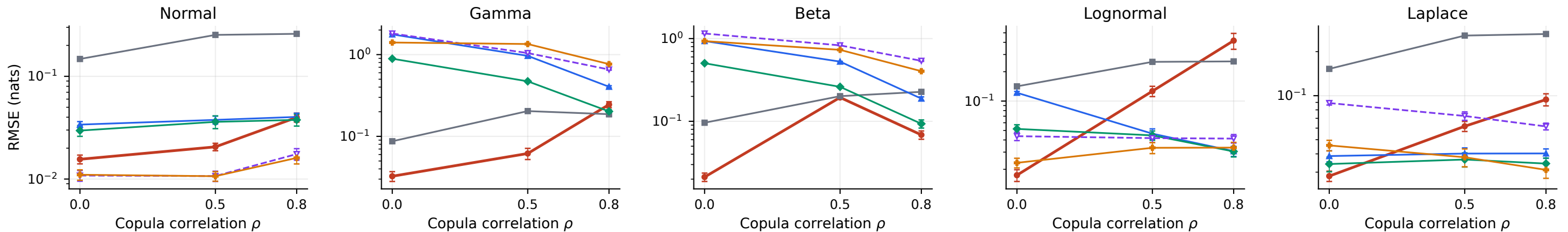
(d) Dependence: n = 20,000, d = 5
