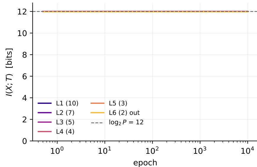
A: tanh at machine precision
