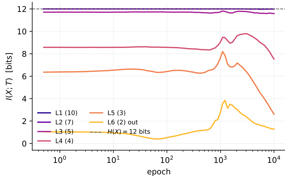
tanh
