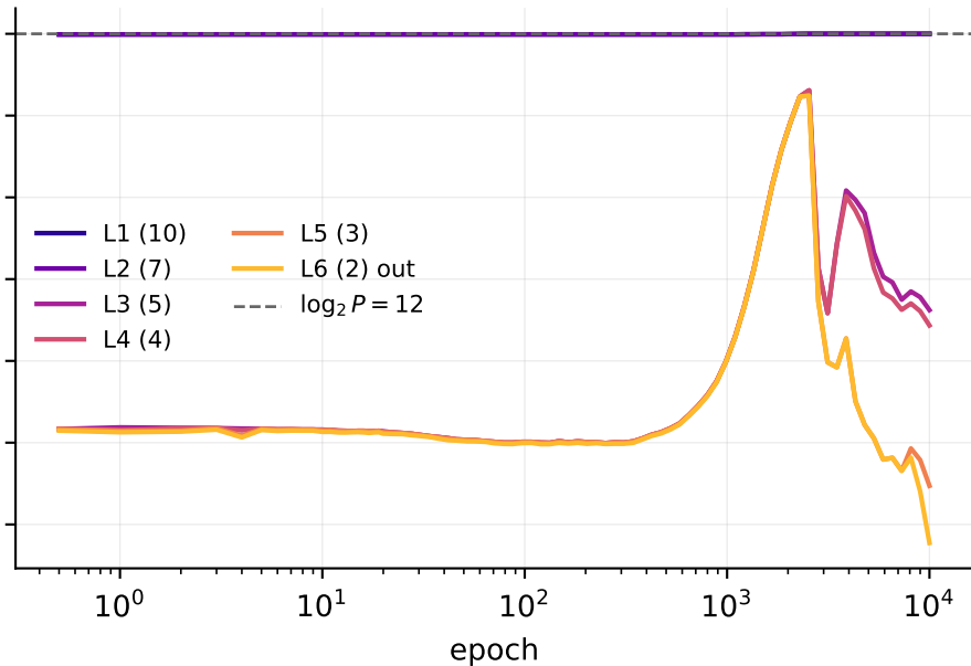
C3 A: ReLU, machine precision
