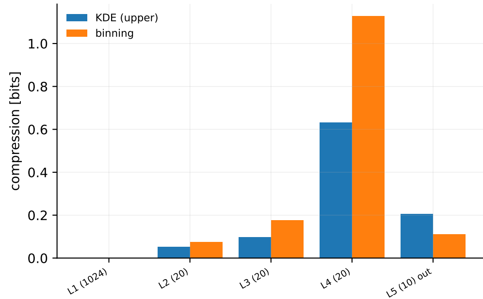
tanh
