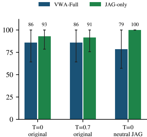
(b) Llama 3.1 8B robustness checks
