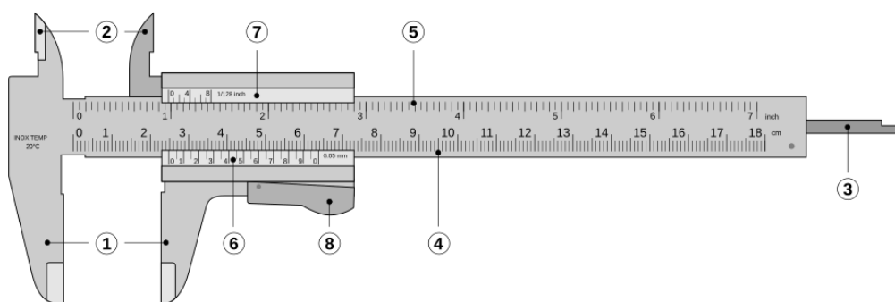
Abbildung 10: Standardmessschieber, (Wikimedia 2023)
