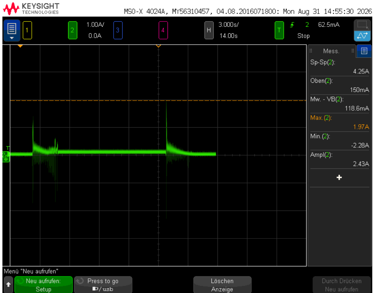
Abbildung 18: Oszilloskop ACT-Motor Fall 7
