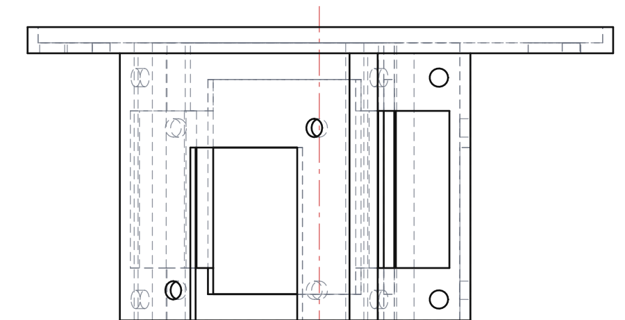
側面図 SIDE
