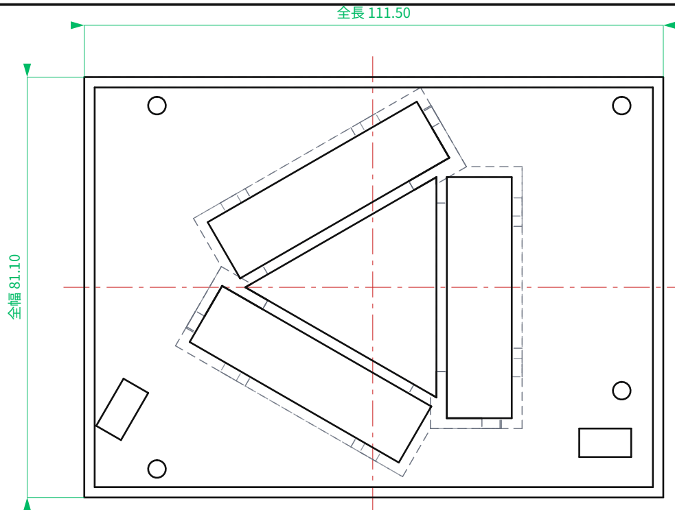
平面図 TOP
