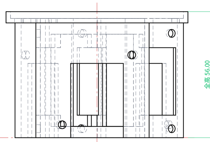
正面図 FRONT
