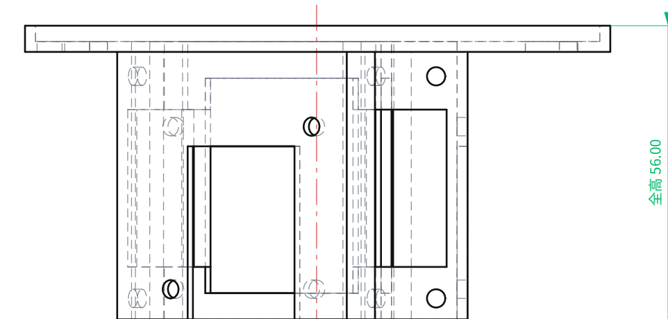
側面図 SIDE
