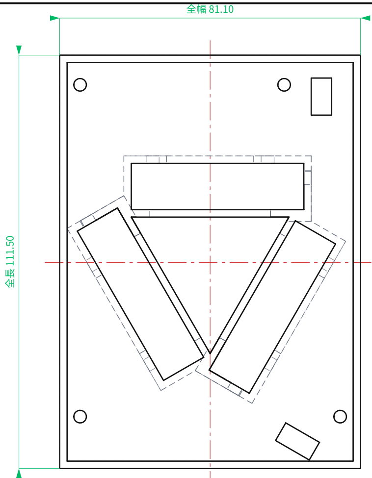
平面図 TOP
