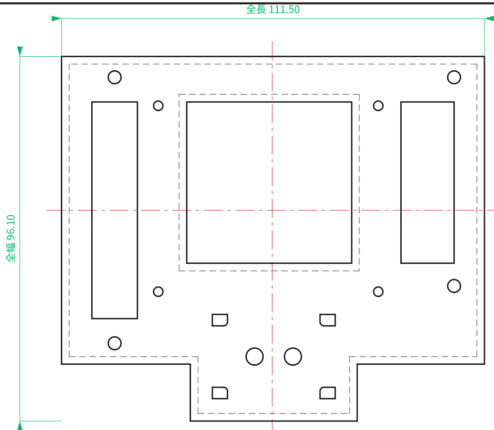
平面図 TOP
