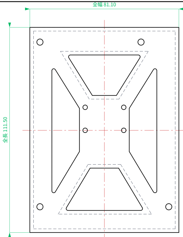
平面図 TOP
