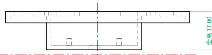
正面図 FRONT
