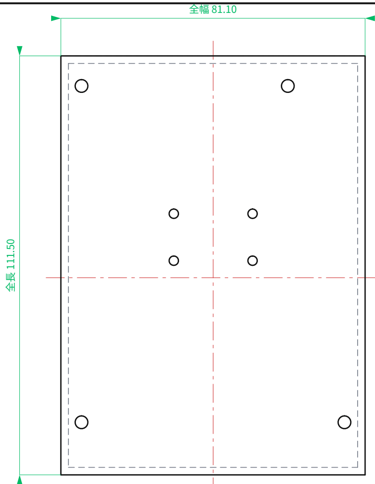
平面図 TOP
