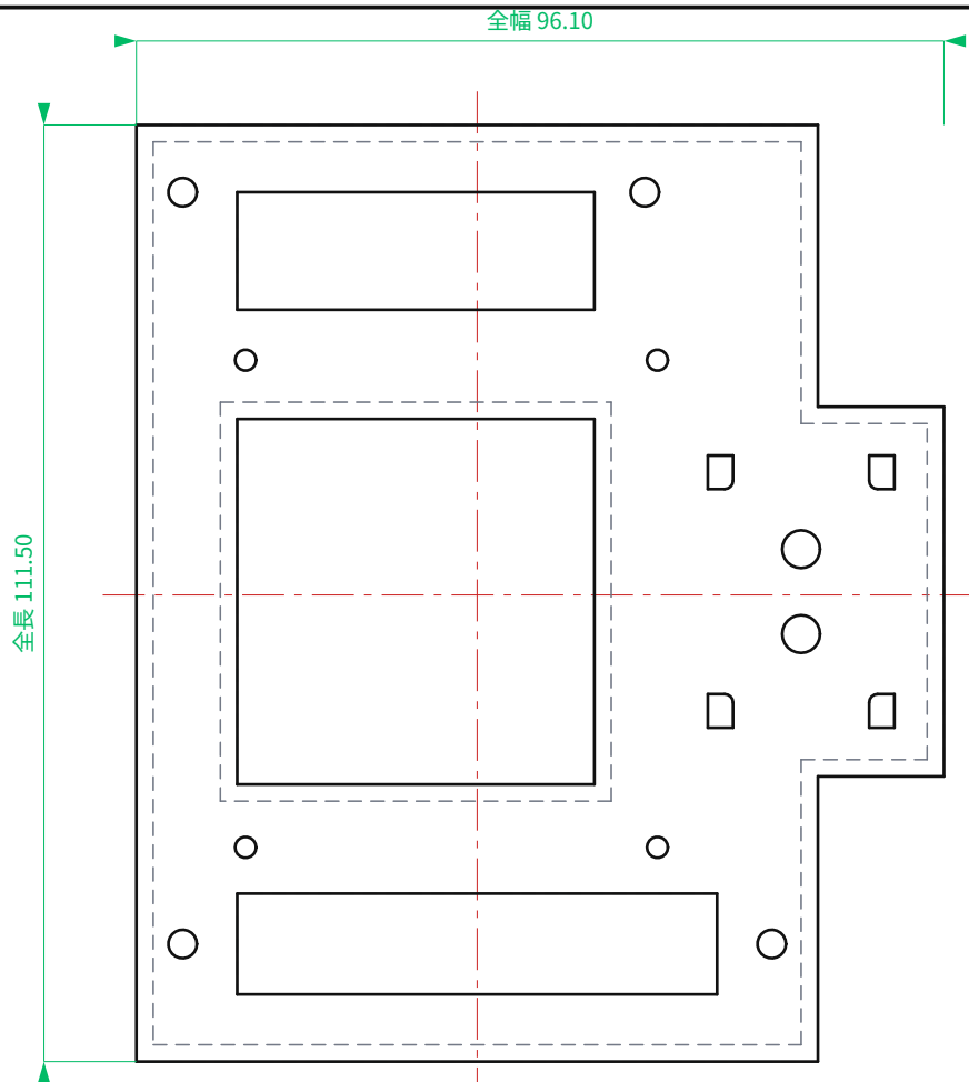
平面図 TOP
