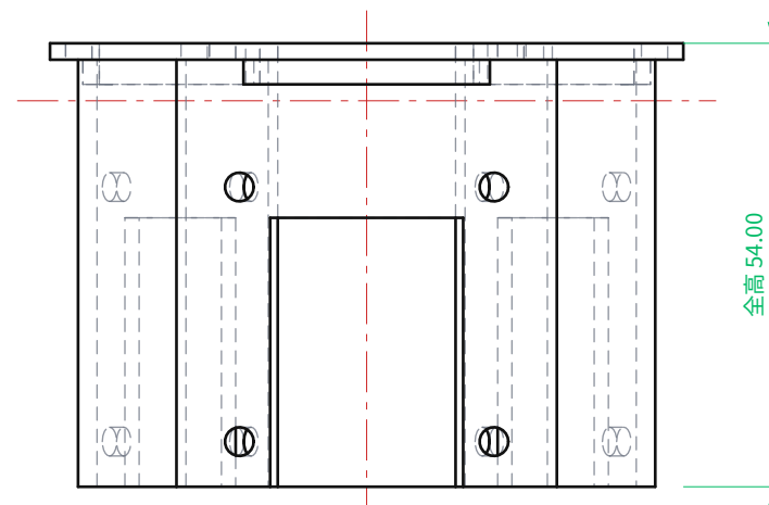
正面図 FRONT
