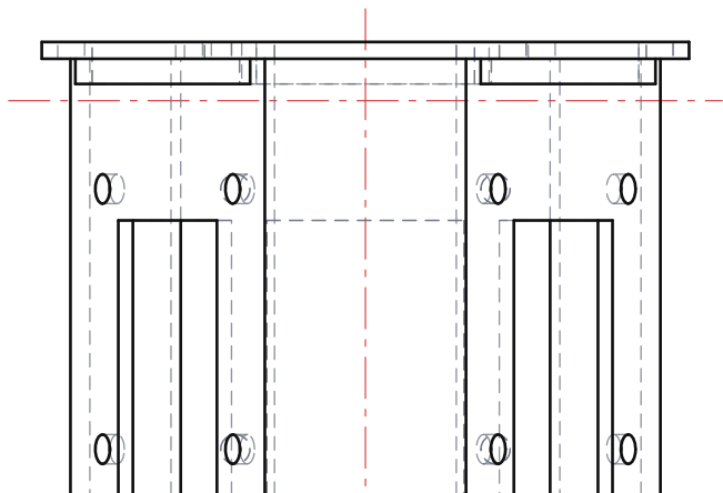
背面図 REAR
