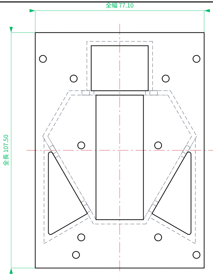
平面図 TOP
