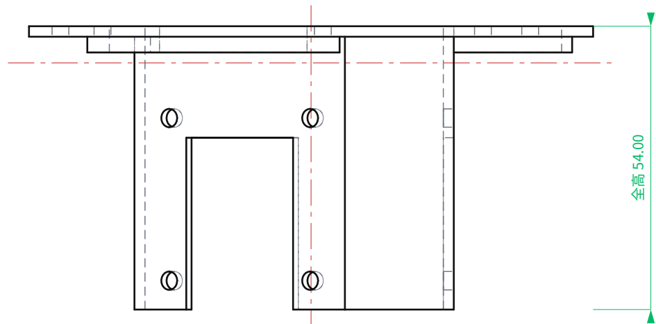
側面図 SIDE
