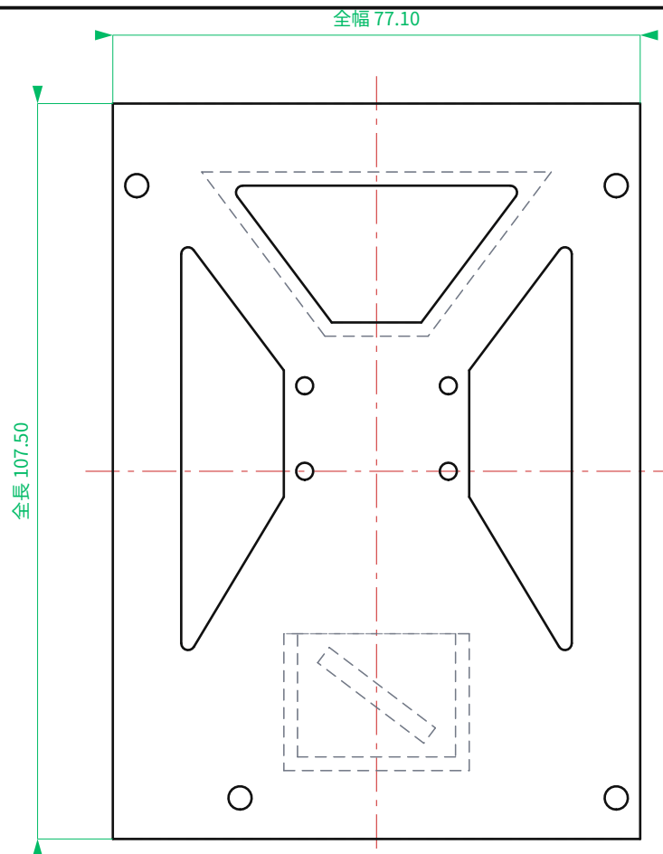
平面図 TOP
