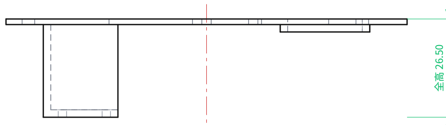
側面図 SIDE
