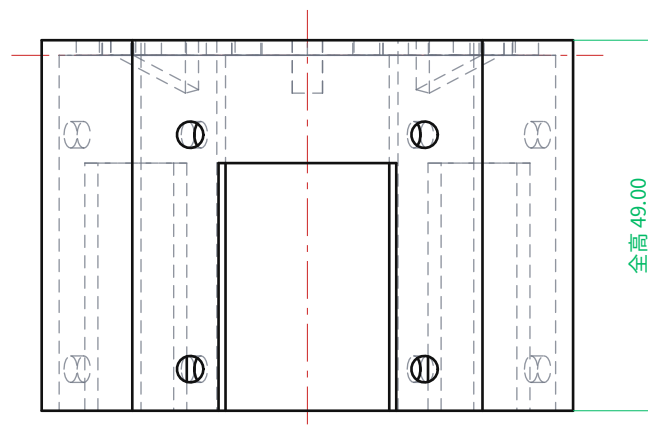
正面図 FRONT
