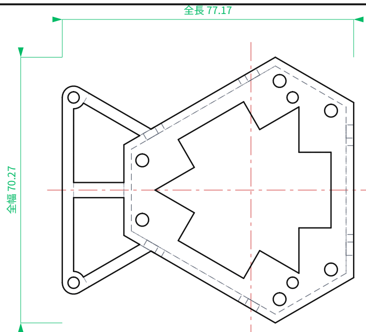
平面図 TOP
