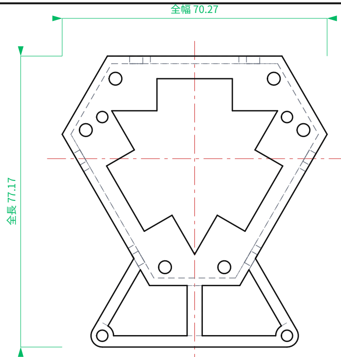
平面図 TOP
