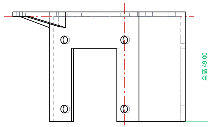
側面図 SIDE
