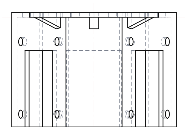
背面図 REAR
