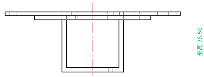
正面図 FRONT
