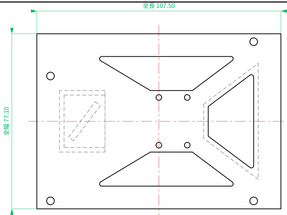
平面図 TOP
