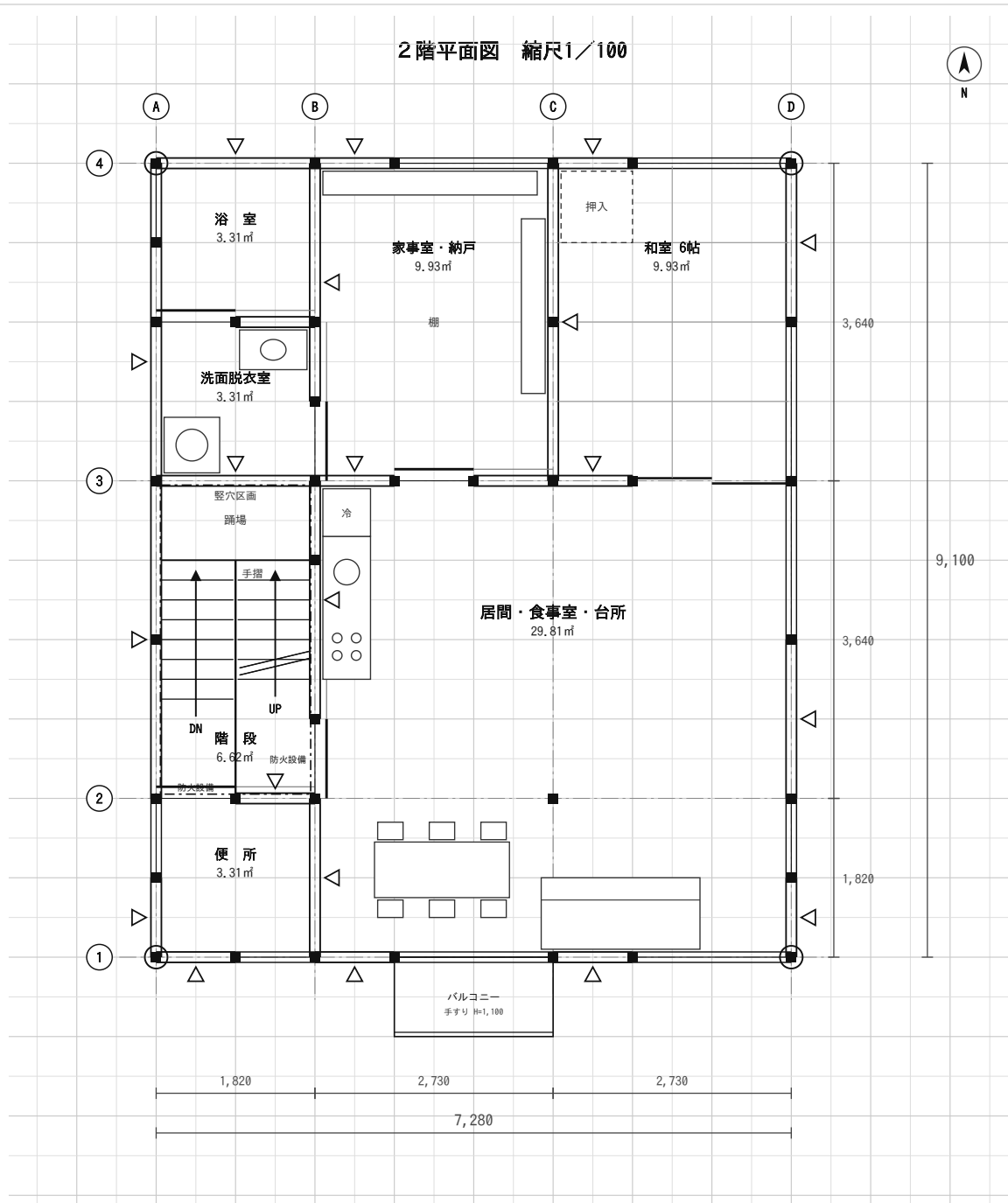
2階平面図。1階と同じ柱・同じ外壁・同じ階段の位置に、住まいの部屋をのせる。
