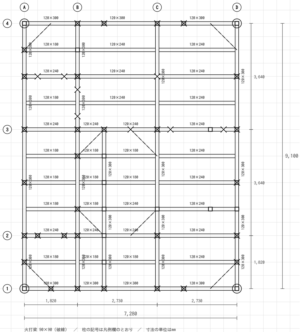
3階床伏図 縮尺1/100
