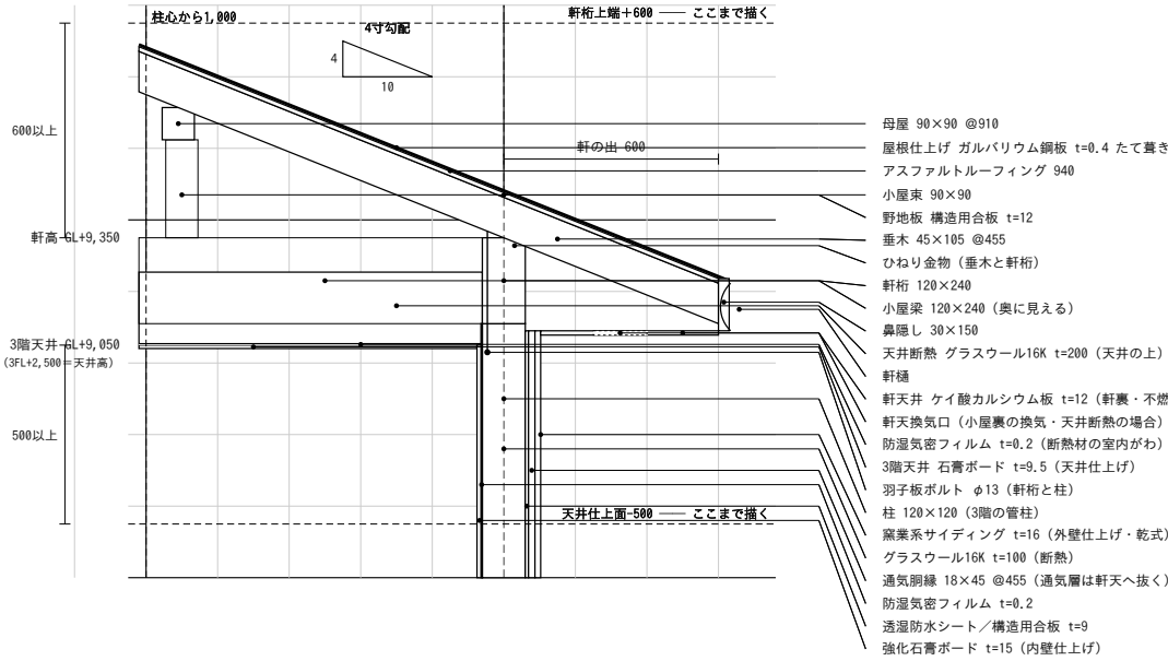
提出する形 部分詳細図（断面）が「軒先まわり」だったとき 縮尺1/20
