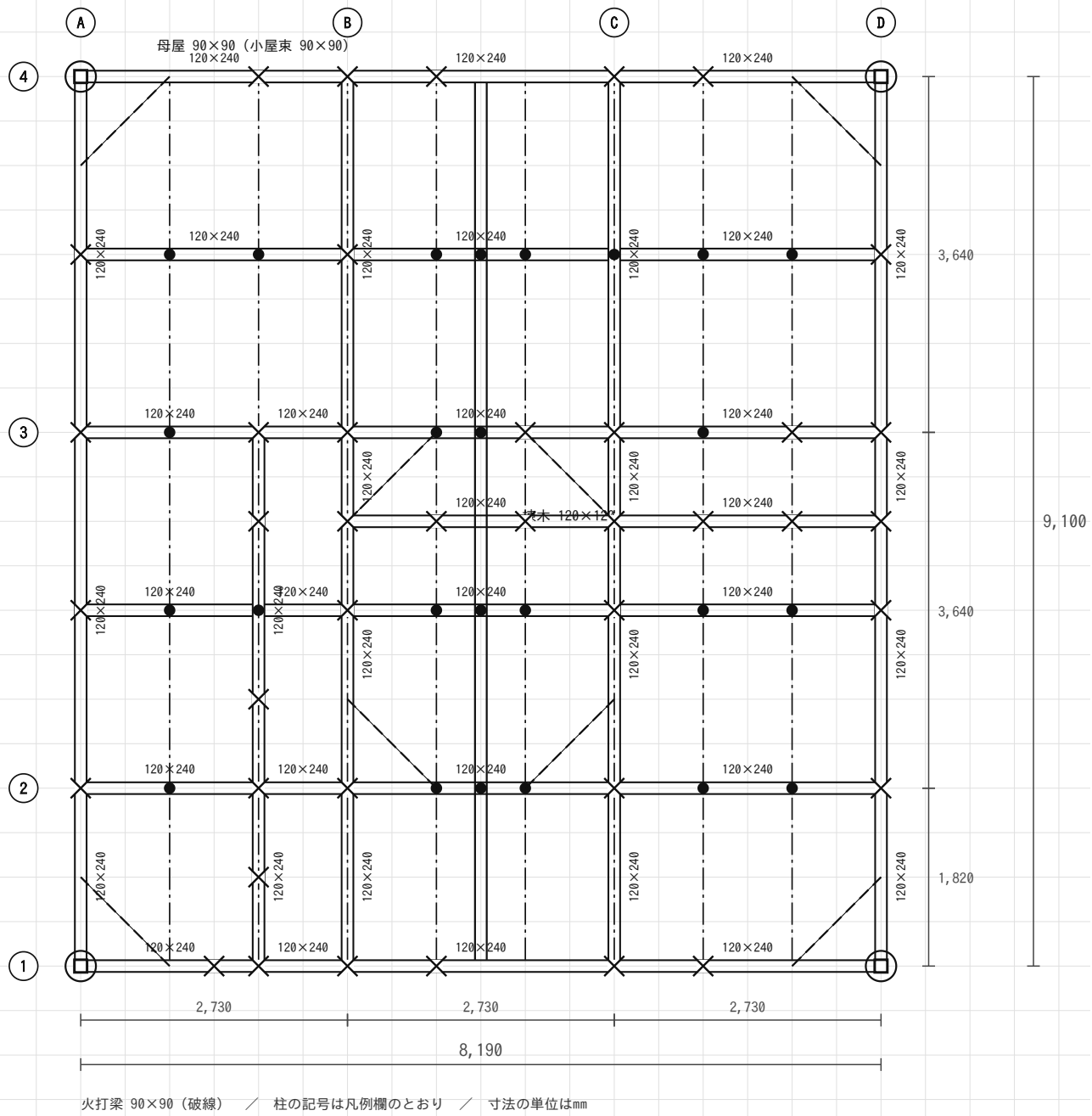
予想問題 B 解答例 小屋伏図 縮尺1/100
