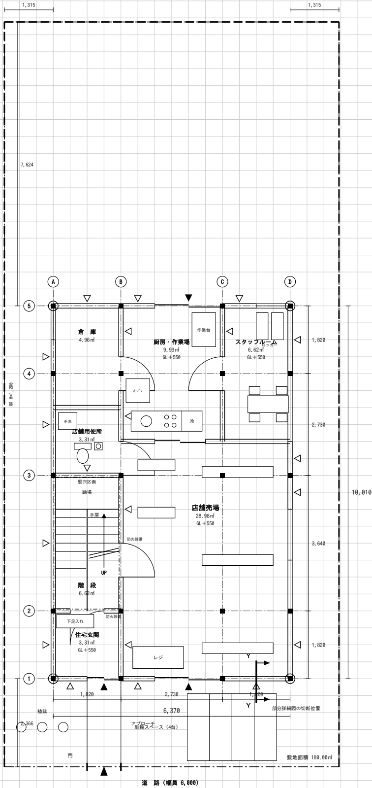
1 階平面図 兼 配置図 縮尺1／100
