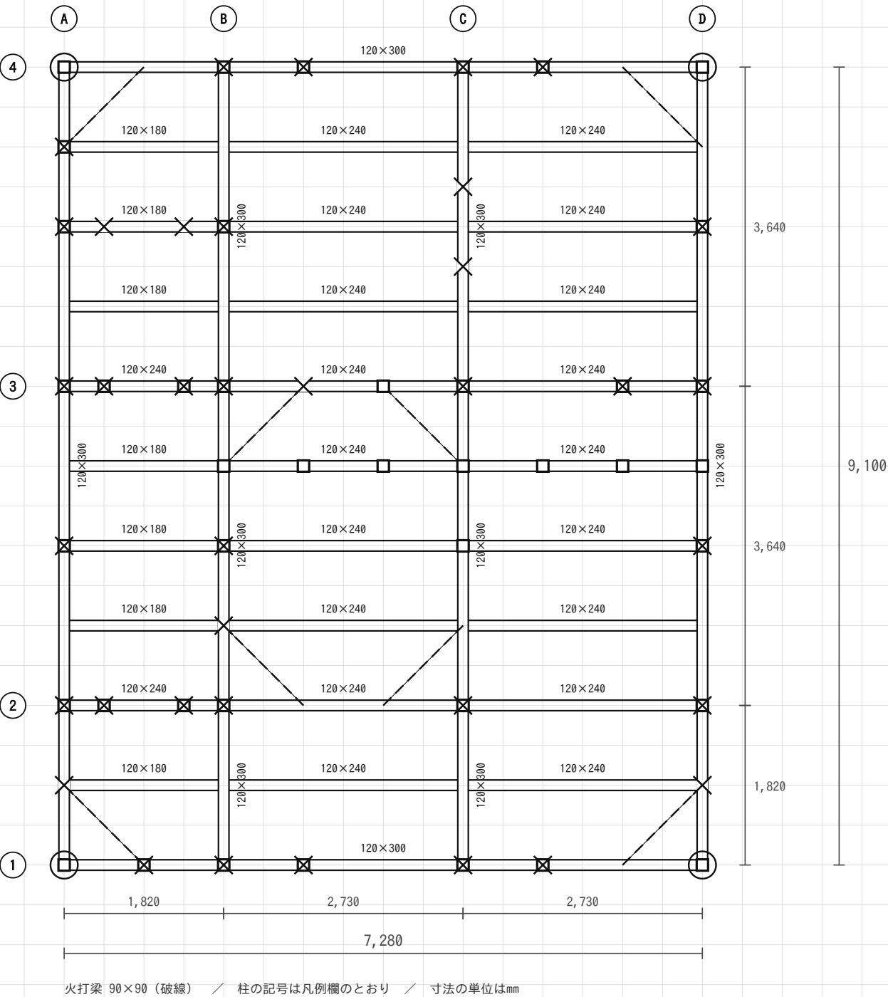
3階床伏図（2階の床も同じ組み方） 縮尺1／100
