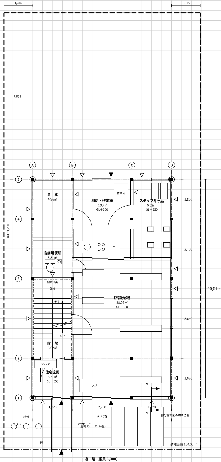
1 階平面図 兼 配置図 縮尺1／100
