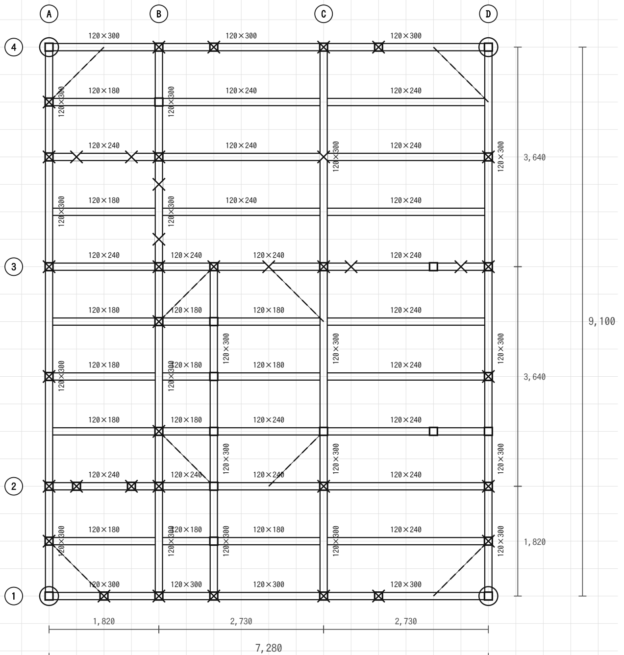
3階床伏図 縮尺1/100
