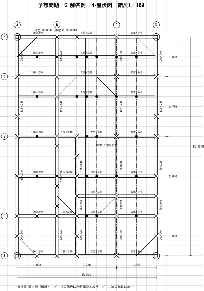
(4) 小屋伏図 (1/100)
