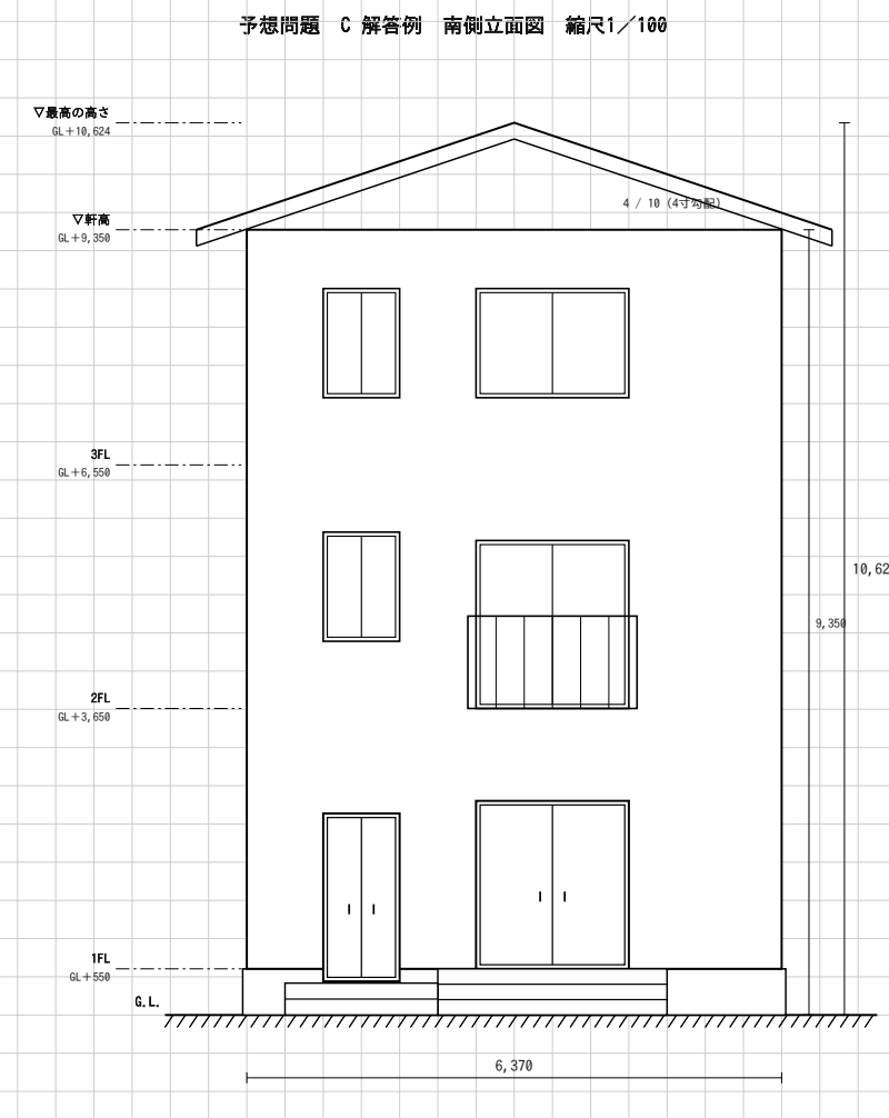
(5) 南側立面図 (1/100)
