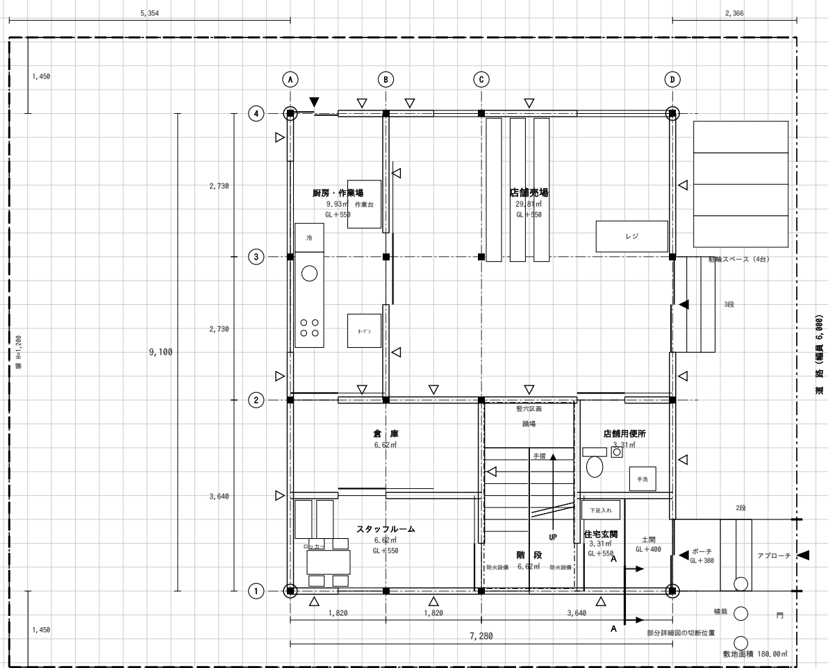
(1) 1 號平面圖兼配置圖 縮尺 1/100
