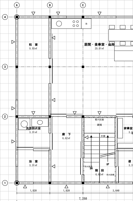
(2) 2階平面図 縮尺1/100
