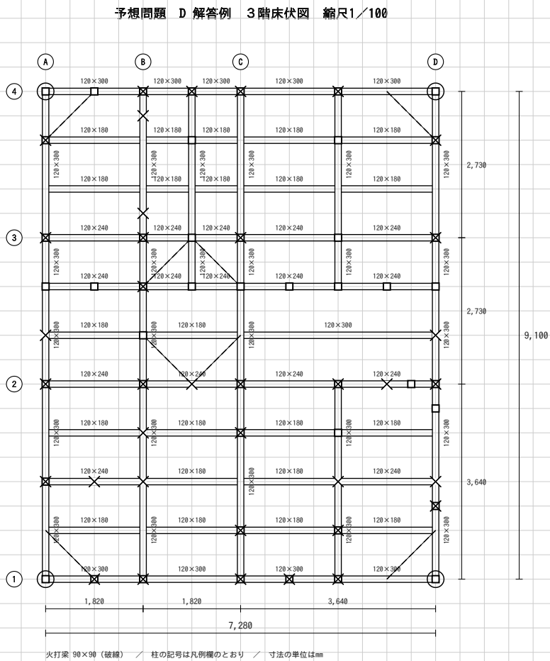
(4) 3階床伏図 (1/100)
