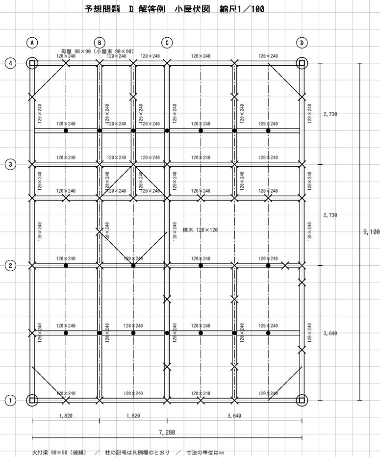
(4) 小屋伏図 (1/100)
