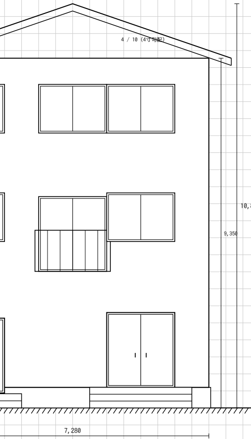
解答例 南側立面図 縮尺1/100
