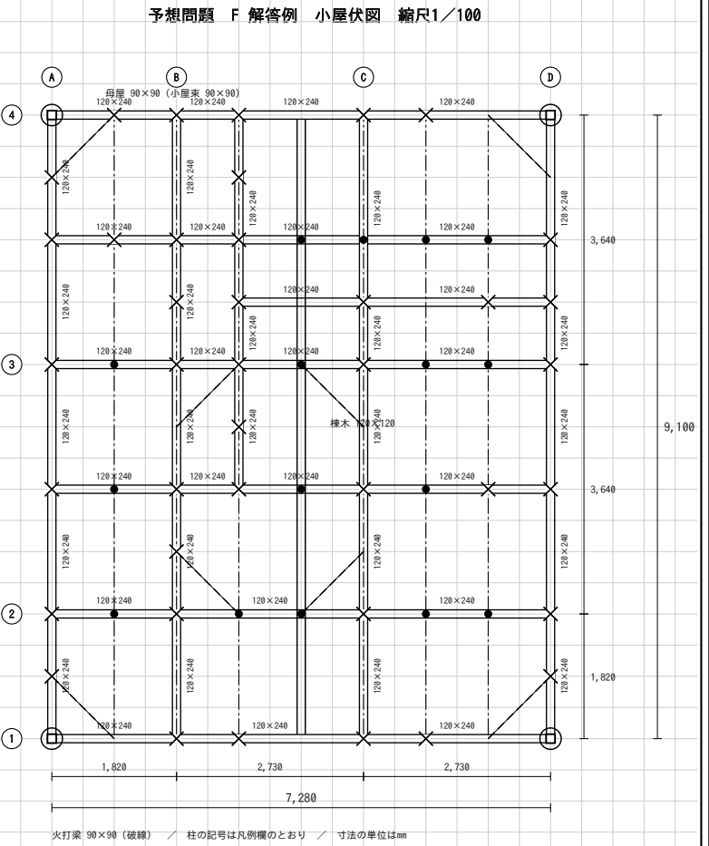
(4) 小屋伏図 (1/100)
