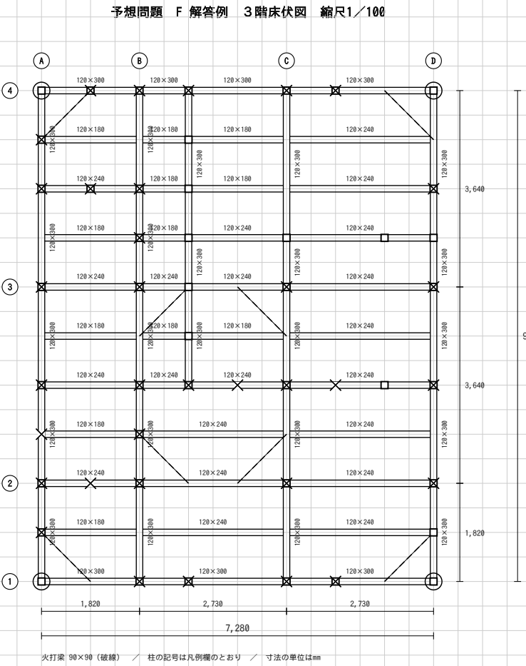
(4) 3階床伏図 (1/100)
