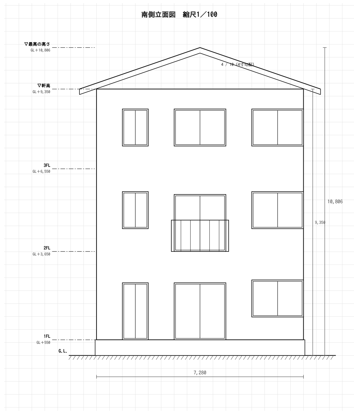
(5) 南側立面図 (1/100)
