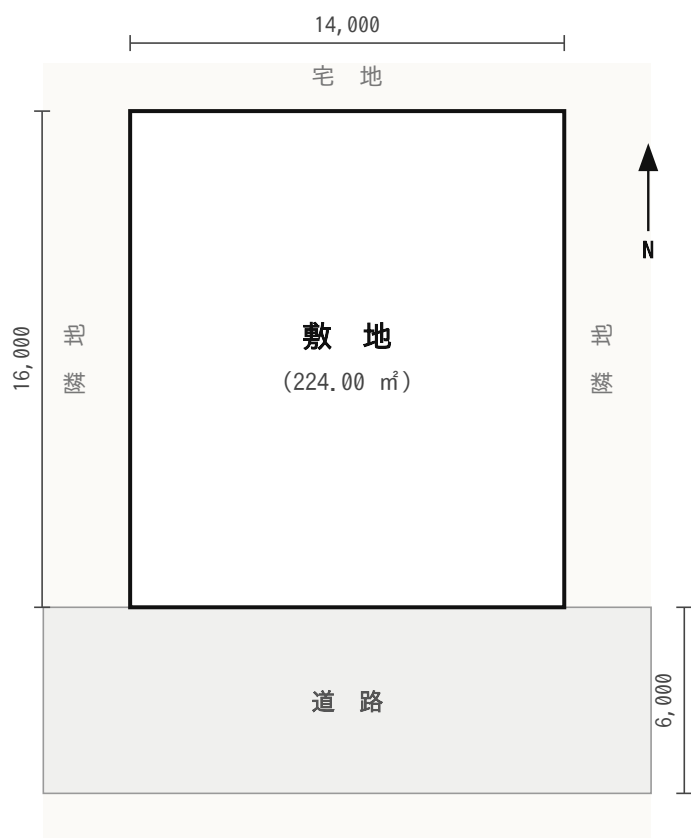
敷地図（縮尺：1/500、単位：mm）
