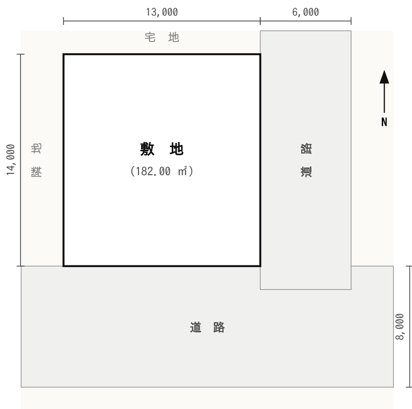
敷地図（縮尺：1/500、単位：mm）
