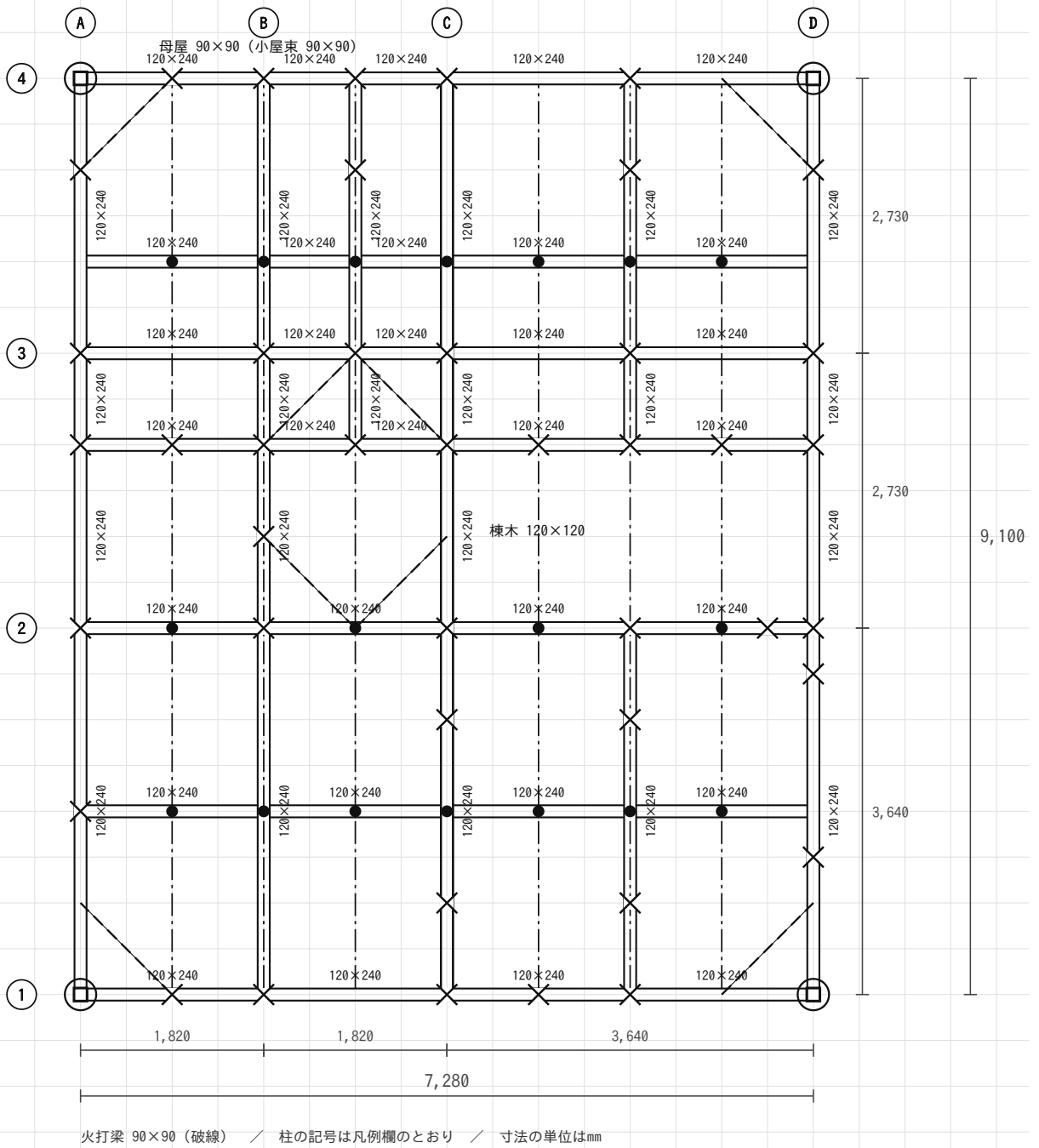
予想問題 D 解答例 小屋伏図 縮尺1/100
