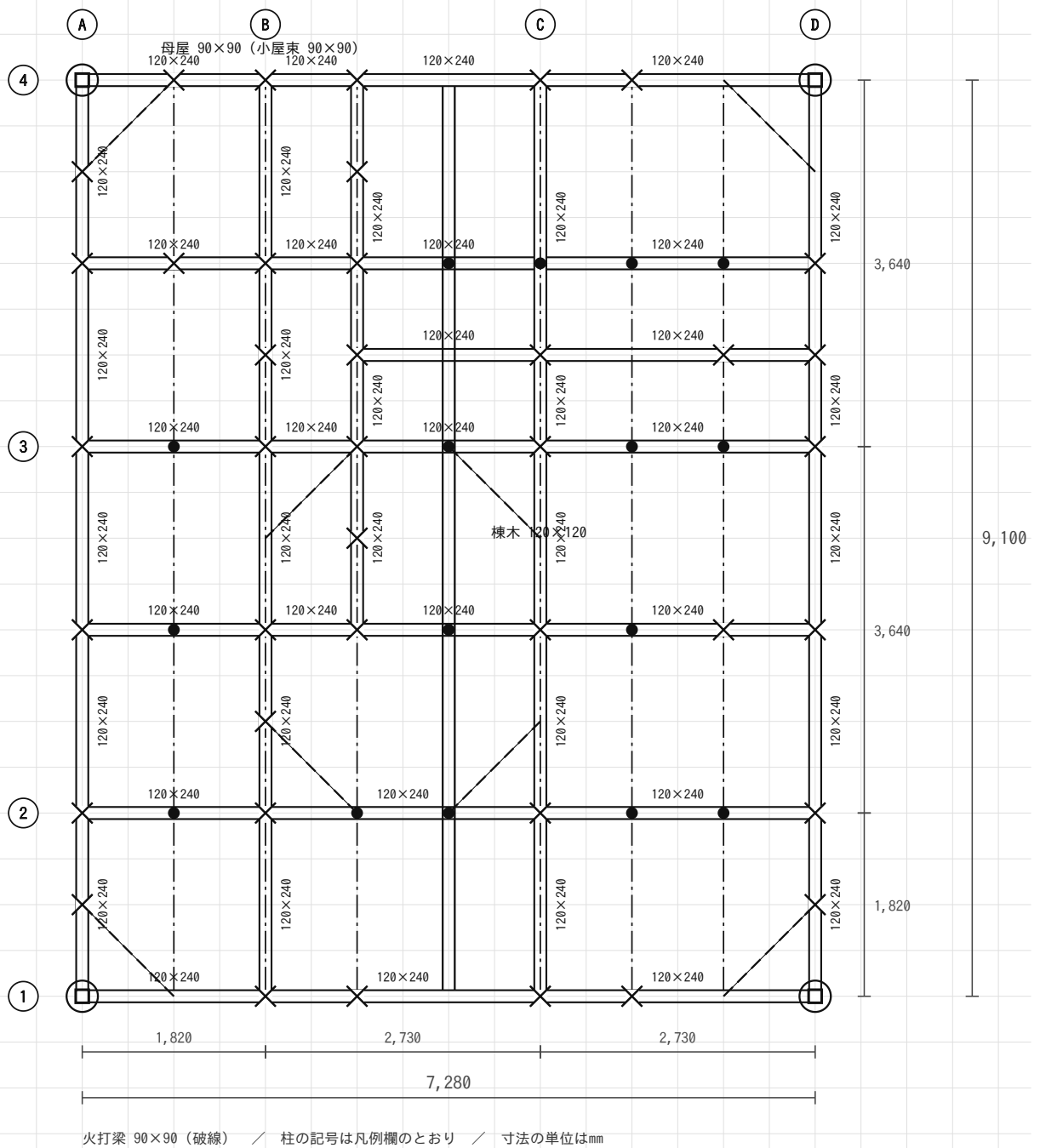
予想問題 F 解答例 小屋伏図 縮尺1/100
