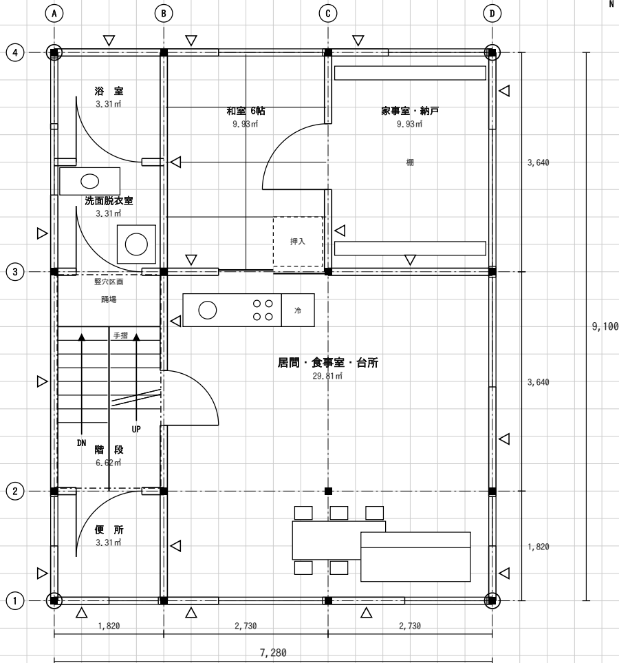
2階平面図 縮尺1／100
