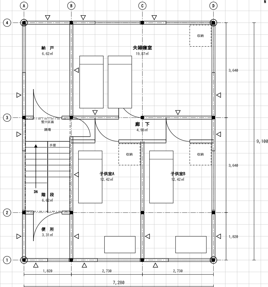
3階平面図 縮尺1／100
