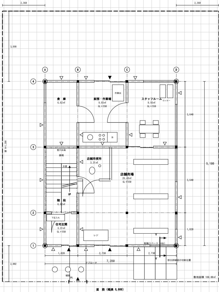
1階平面図 兼 配置図 縮尺1／100
