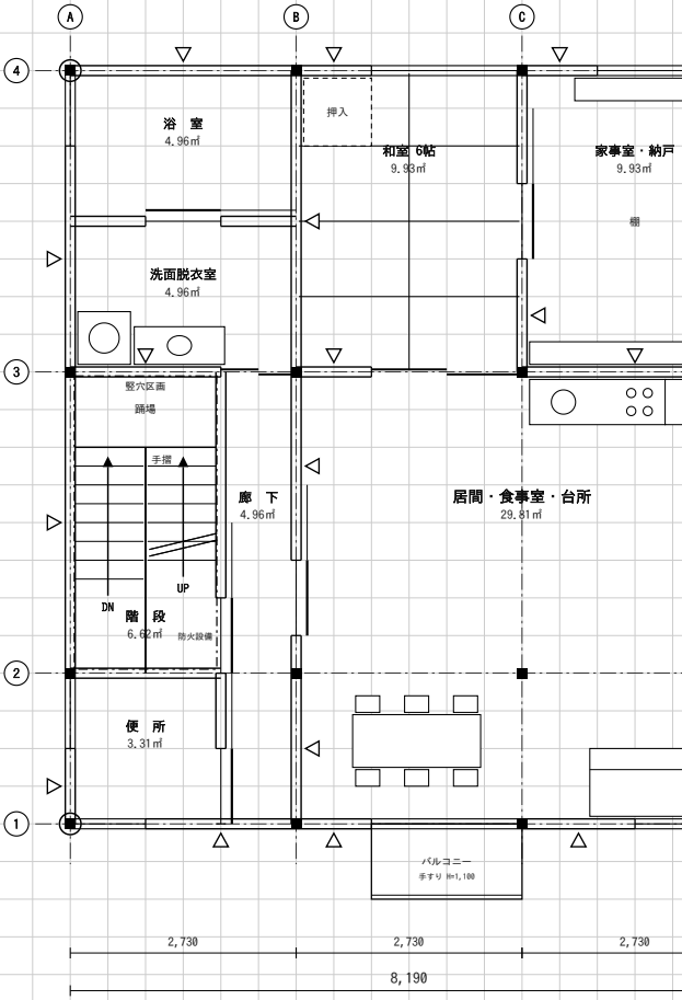
(2) 2階平面図 縮尺1/100
