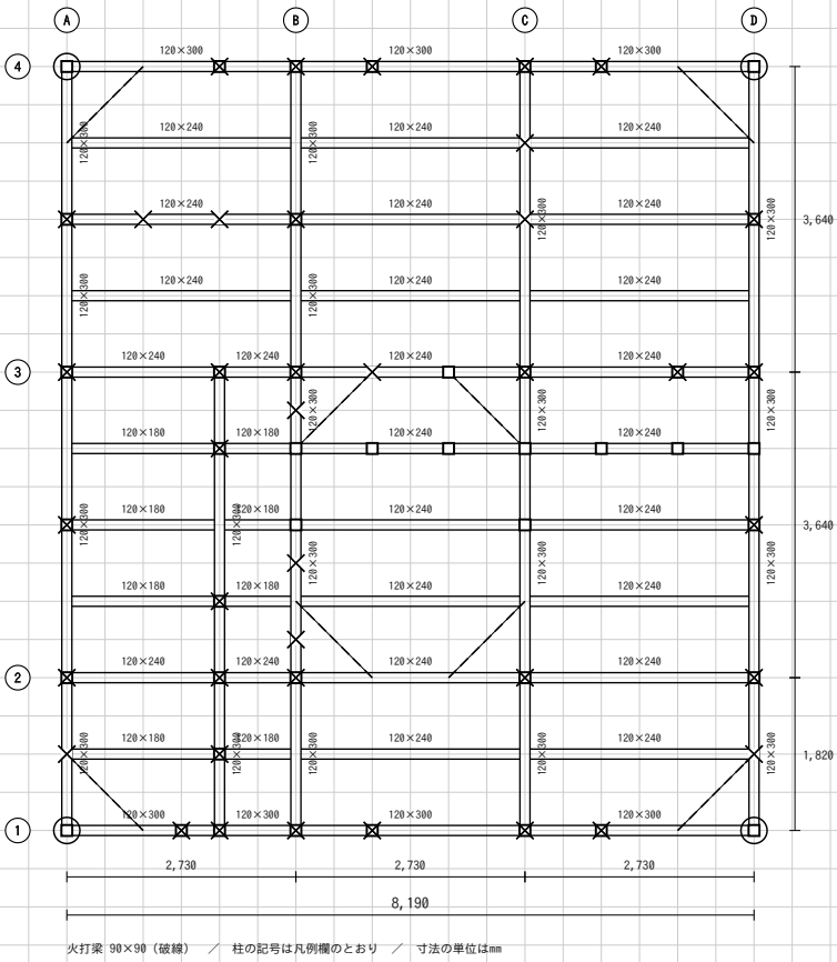
予想問題 B 解答例 3階床伏図 縮尺1/100
