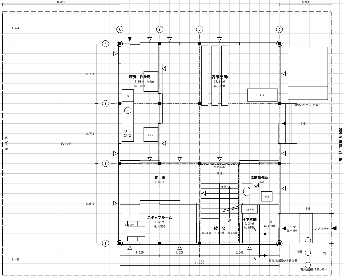
(1) 1階平面図 兼 配置図 縮尺1／100
