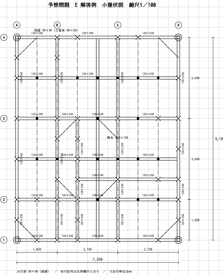
(4) 小屋伏図 (1/100)
