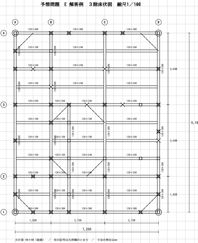
(4) 3階床伏図 (1/100)
