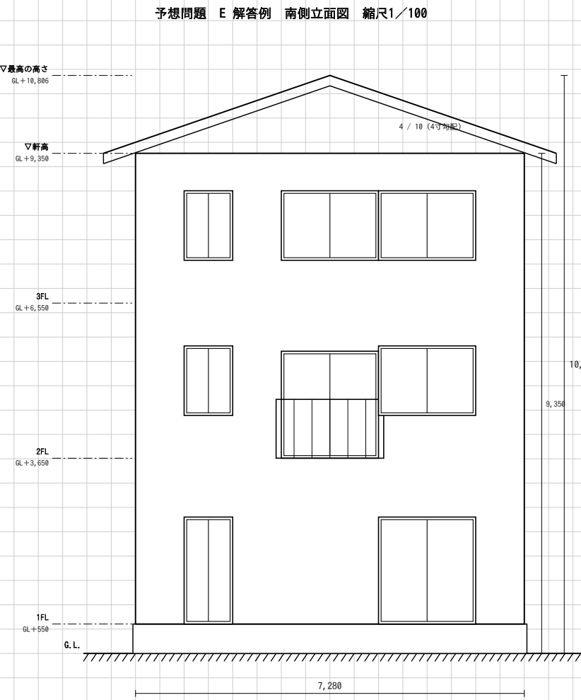
(5) 南側立面図 (1/100)
